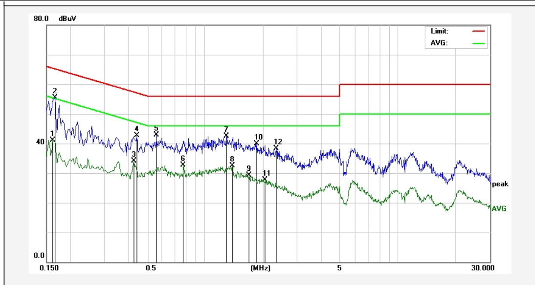
TM3 / Line: Line / Band: 5725-5850 MHz / BW: 20 / CH: M
