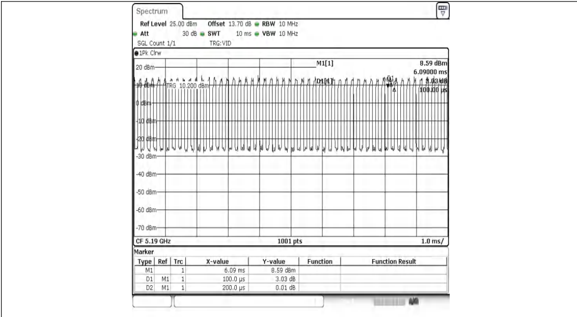
NTNV-11N40MIMO-Ant1-5190
