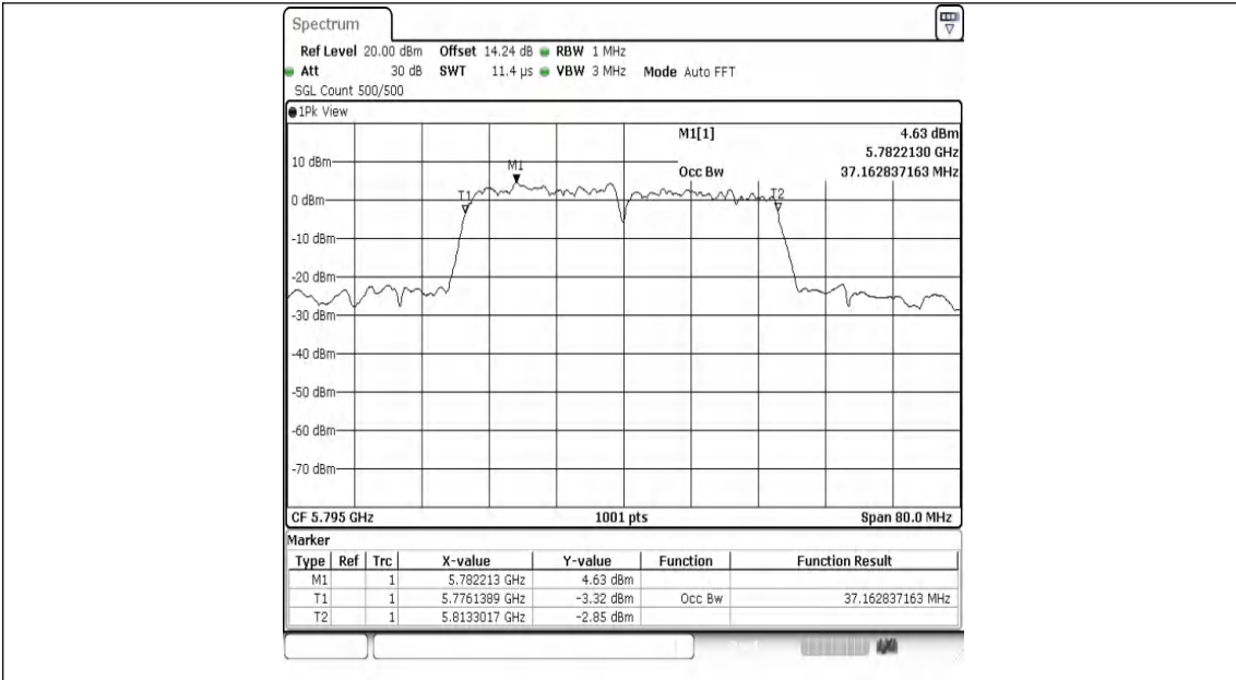
11AC40MIMO-Ant1-5795
