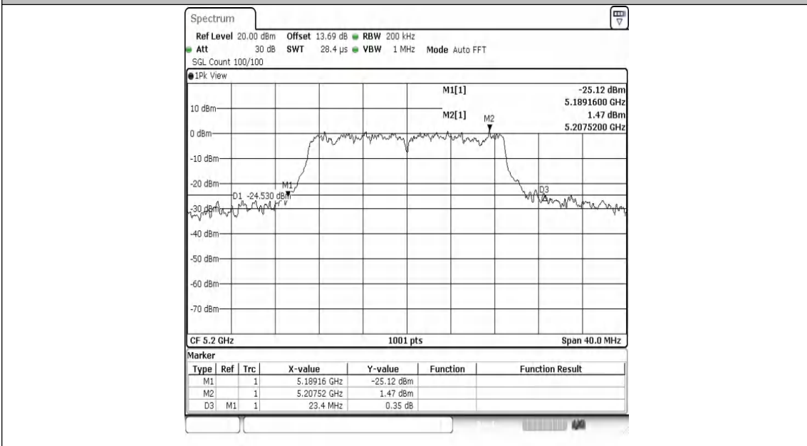
11N20MIMO-Ant2-5200
