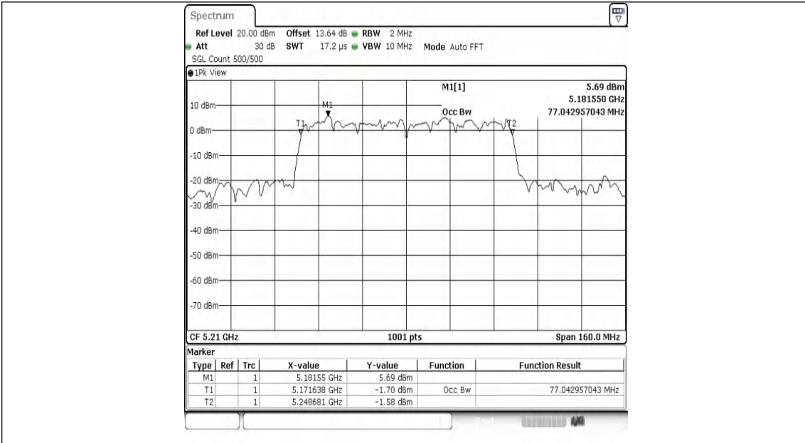
11AC80MIMO-Ant1-5210
