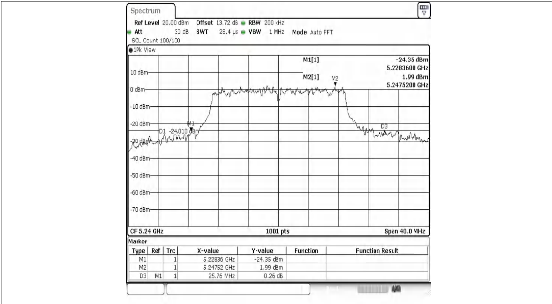
11N20MIMO-Ant1-5240
