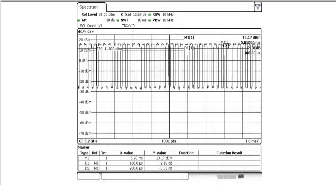
NTNV-11N20MIMO-Ant2-5200
