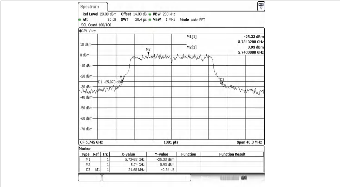
11N20MIMO-Ant1-5745
