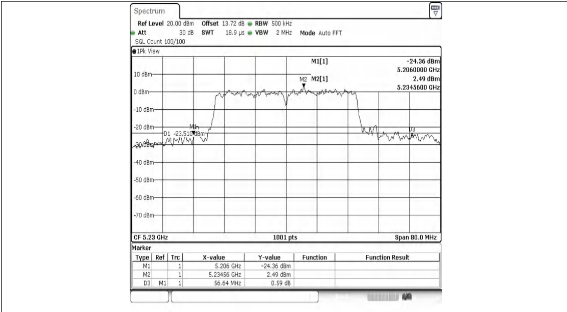
11N40MIMO-Ant1-5230
