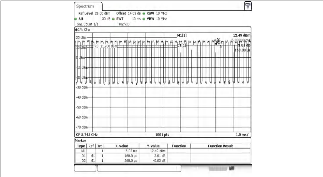
NTNV-11N20MIMO-Ant1-5745
