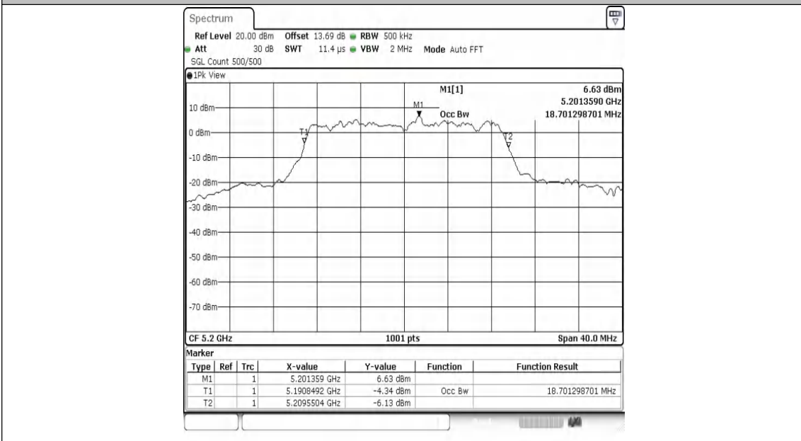
11N20MIMO-Ant2-5200
