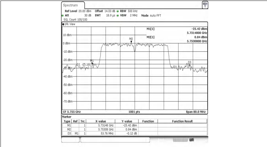
11N40MIMO-Ant1-5755
