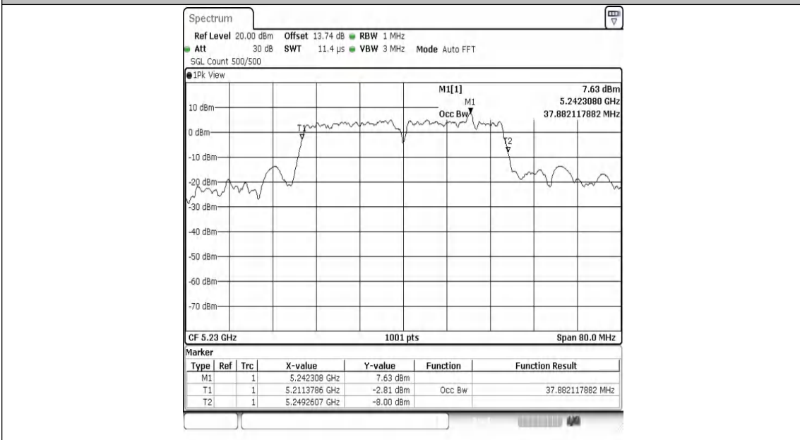
11N40MIMO-Ant2-5230
