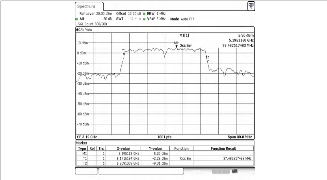
11N40MIMO-Ant1-5190
