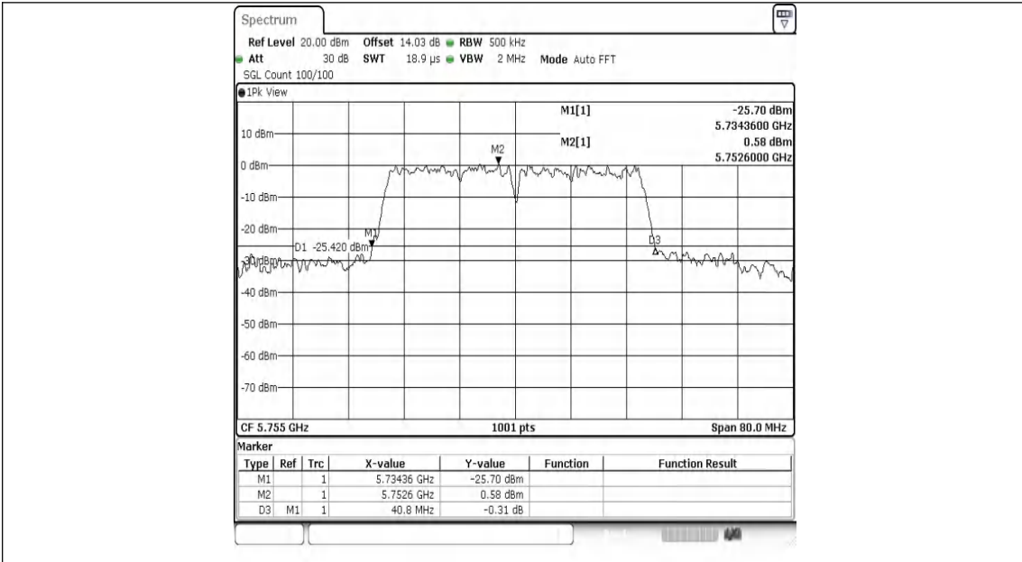
11AC40MIMO-Ant1-5755
