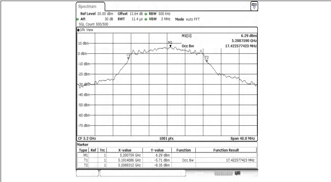
11A-Ant1-5200
