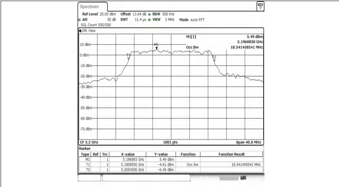
11N20MIMO-Ant1-5200
