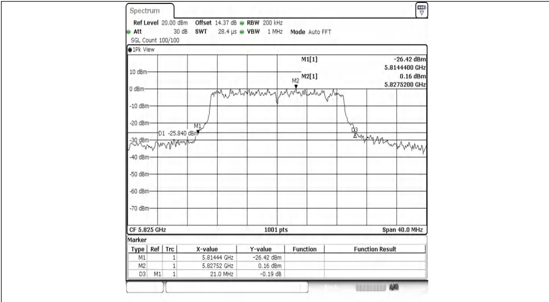
11N20MIMO-Ant1-5825
