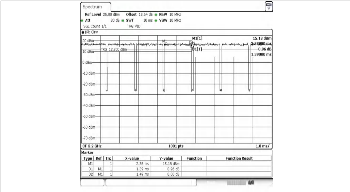
NTNV-11A-Ant1-5200
