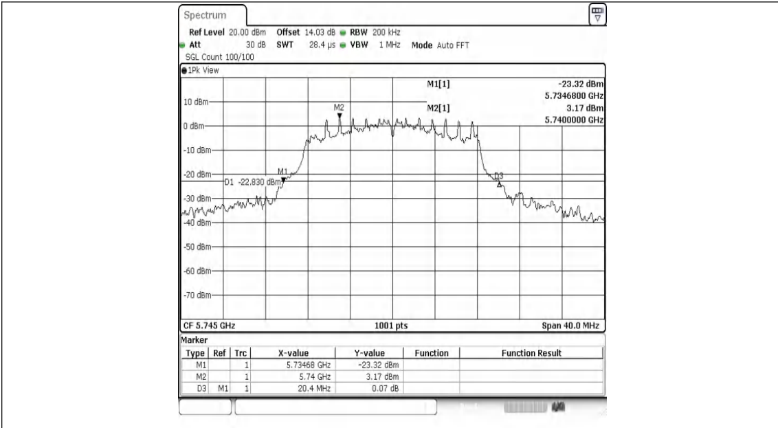
11A-Ant1-5745
