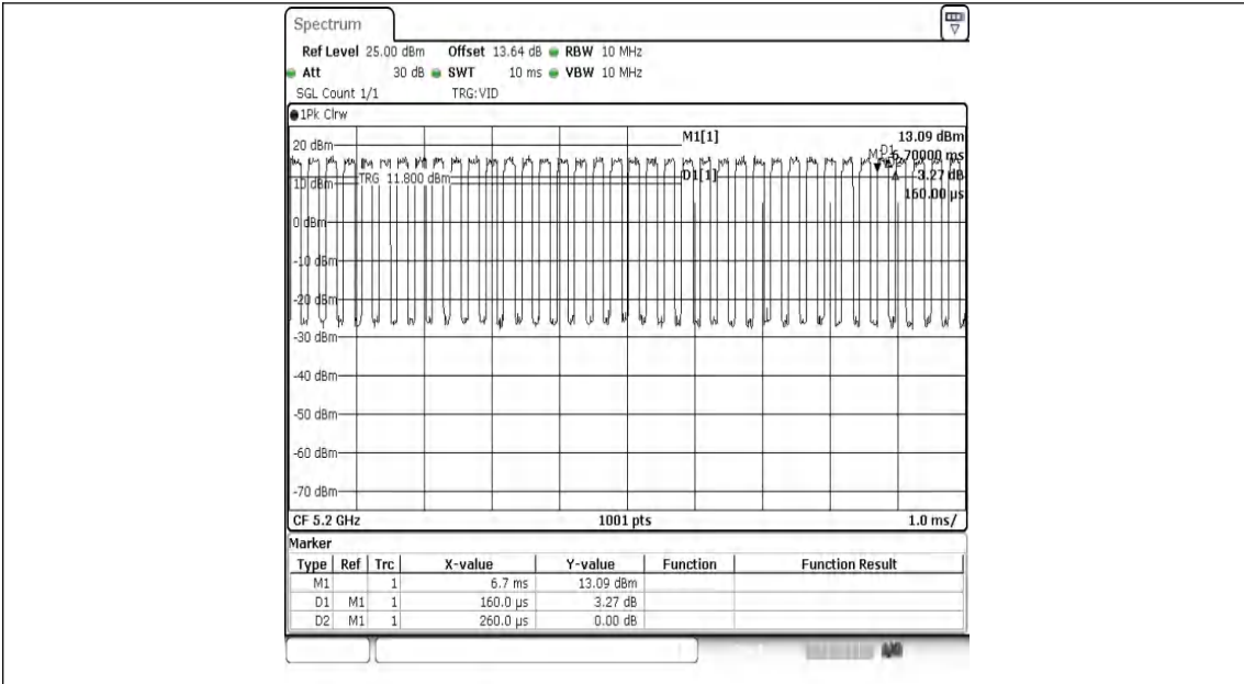
NTNV-11N20MIMO-Ant1-5200
