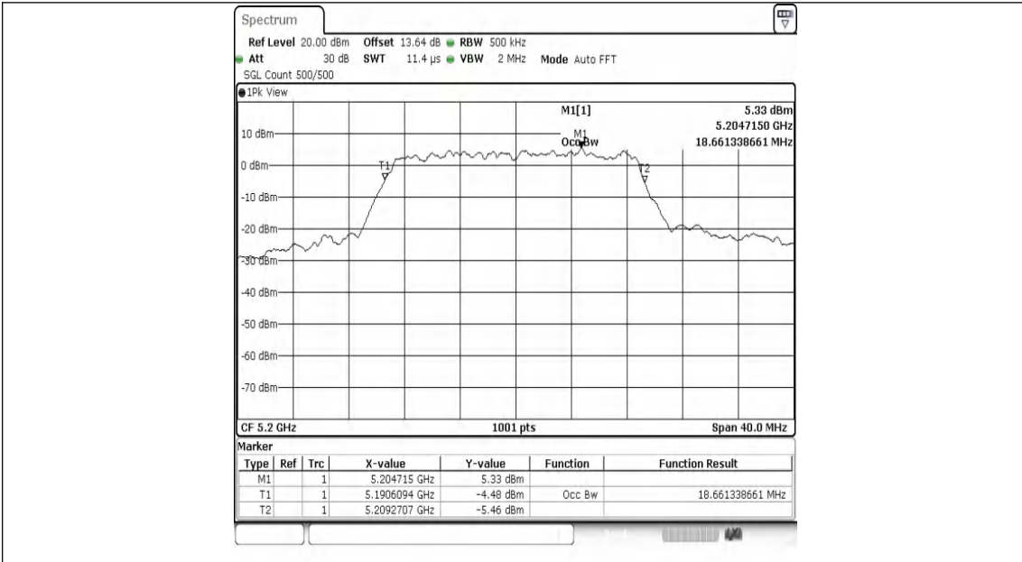
11AC20MIMO-Ant1-5200
