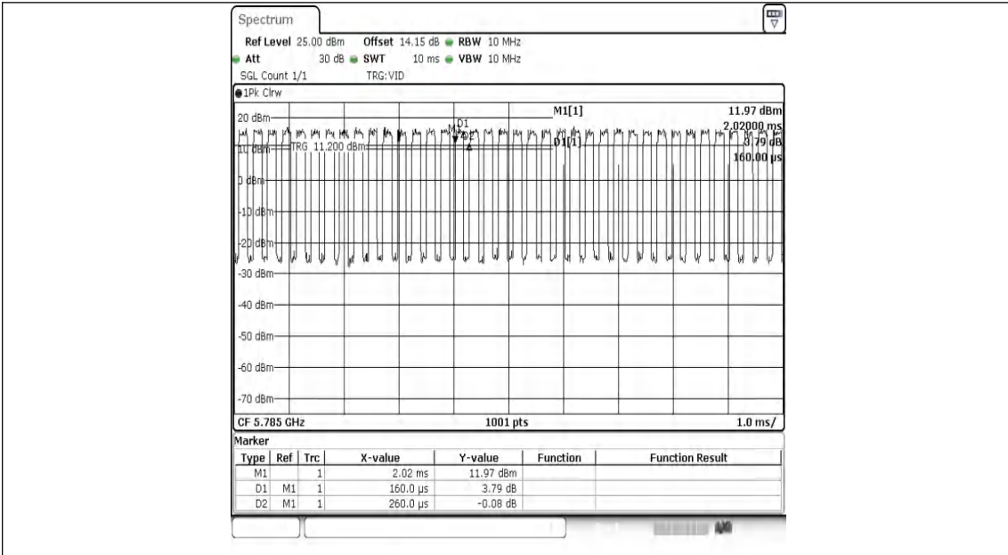
NTNV-11N20MIMO-Ant1-5785
