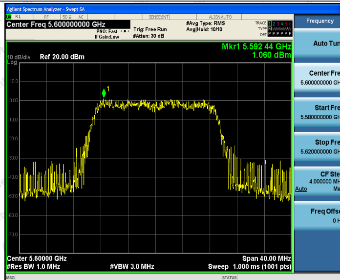
11N20SISO_Ant2_5600
