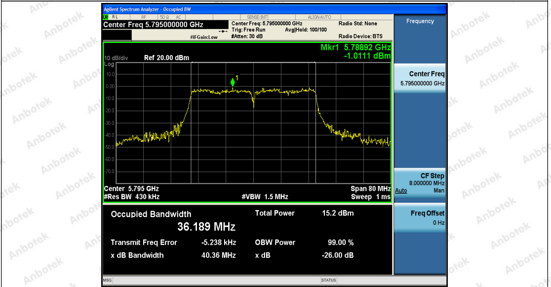
11N40SISO_Ant2_5795
