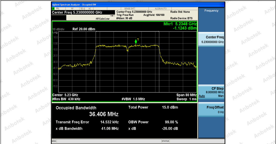
11N40SISO_Ant2_5230
