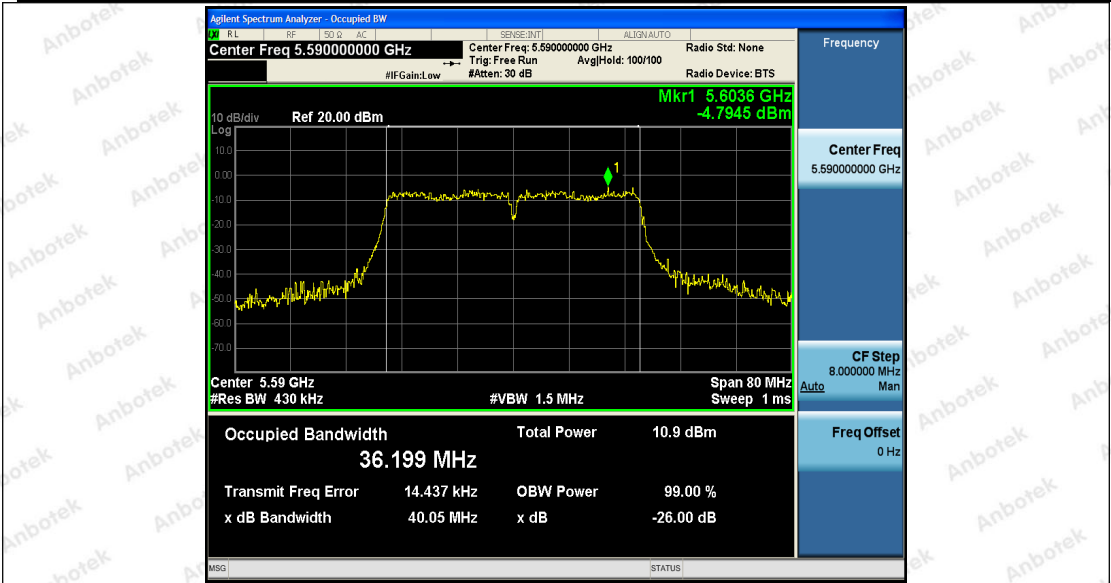
11N40SISO_Ant2_5590
