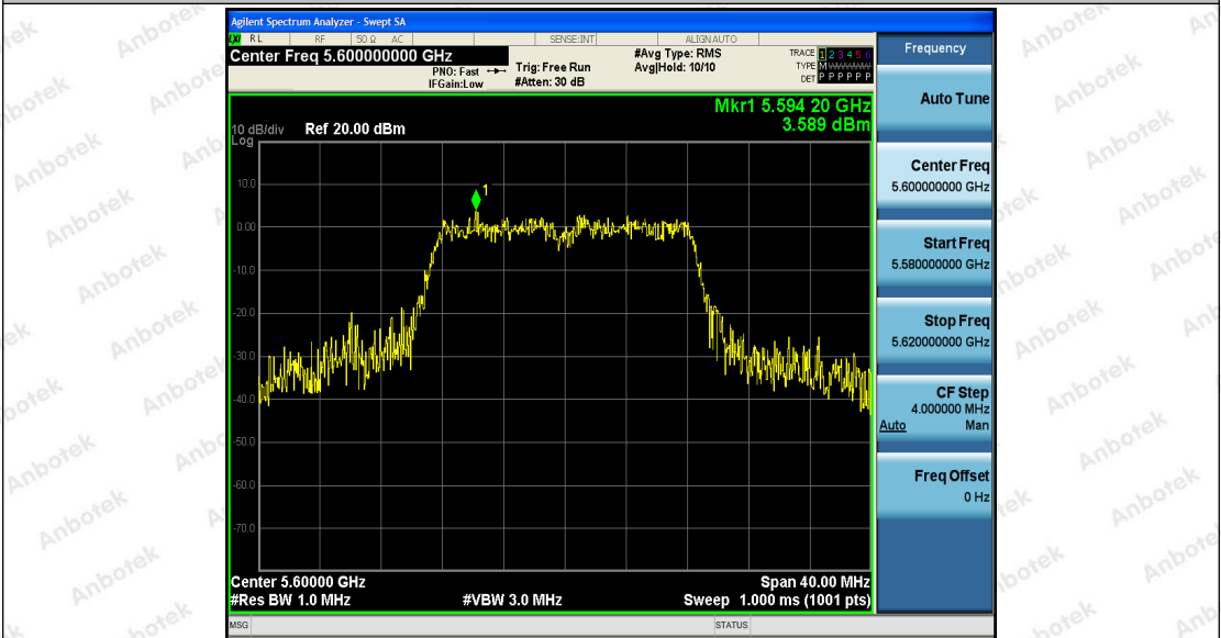
11A_Ant2_5600
