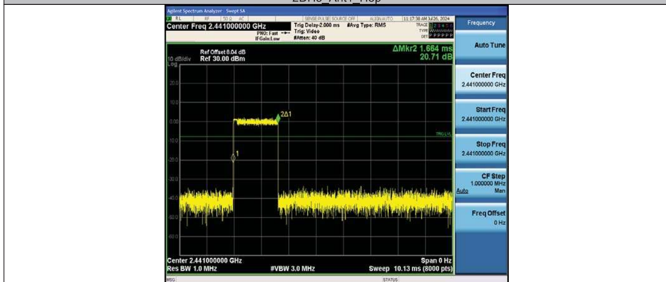
2DH3_Ant1_Hop
