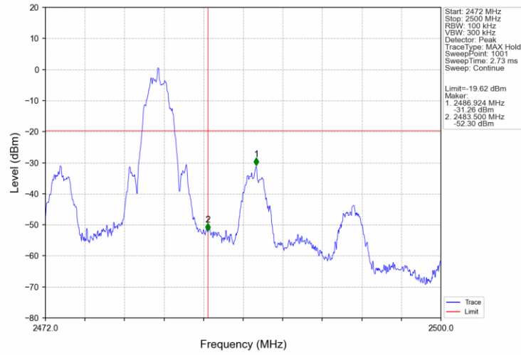
2M_HCH_2480MHz_Ant1_NTNV
