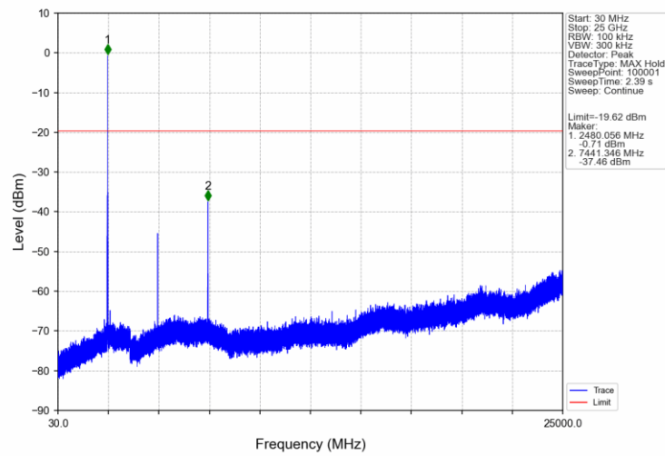
2M_HCH_2480MHz_Ant1_NTNV
