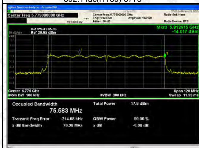
802.11ac(HT80)-5775
