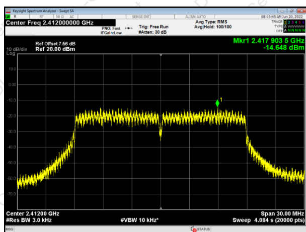
2412MHz
