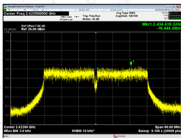
2422MHz
