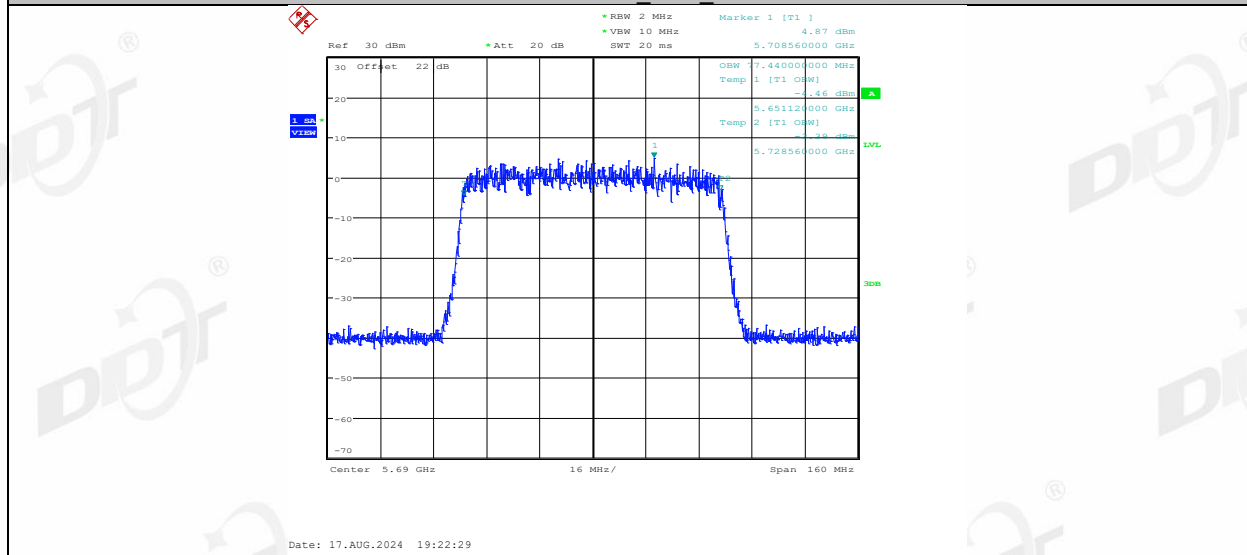
11AX80MIMO_Ant2_5690
