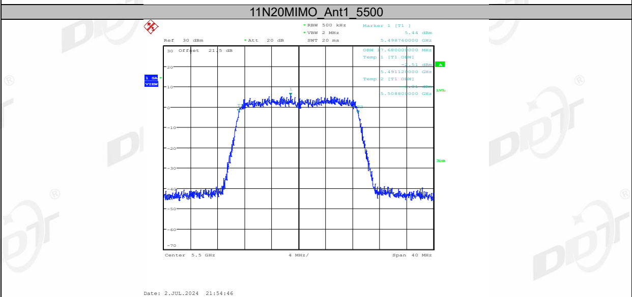
11N20MIMO_Ant2_5500
