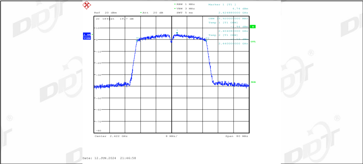
11N40MIMO_Ant2_2422
