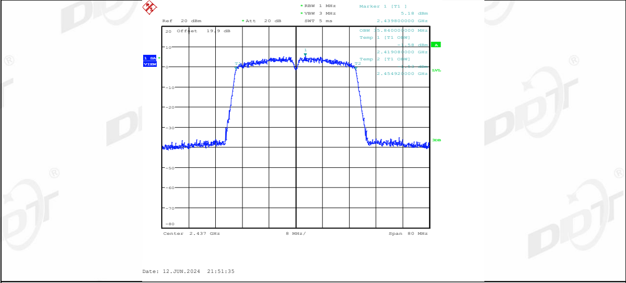
11N40MIMO_Ant2_2437
