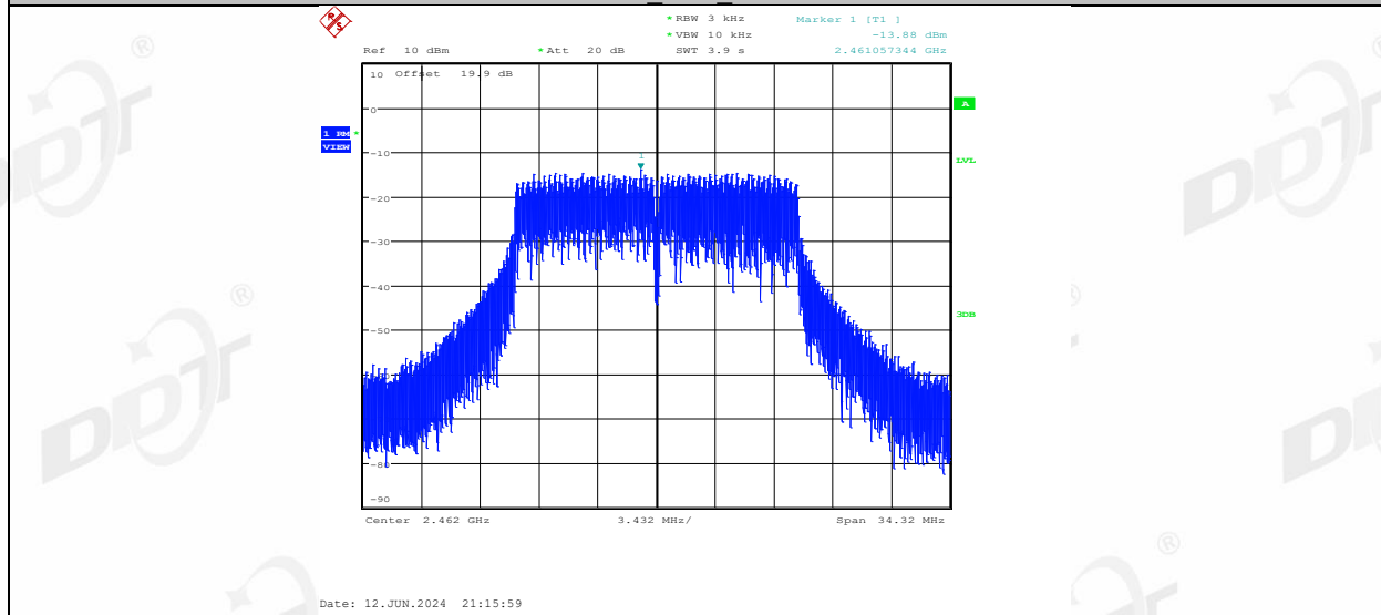
11G_Ant2_2462
