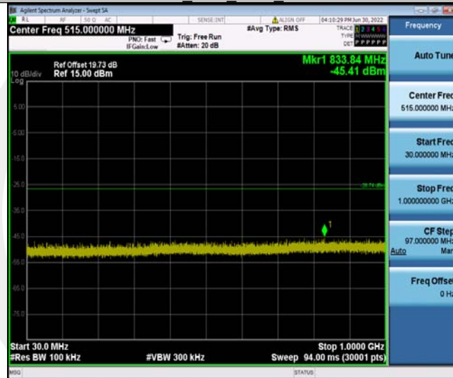
11N20MIMO_Ant2_2462_30~1000
