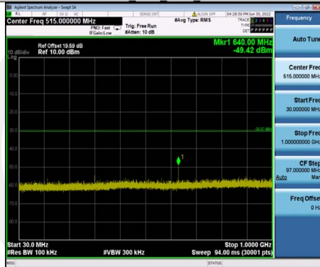
11N40MIMO_Ant2_2422_30~1000
