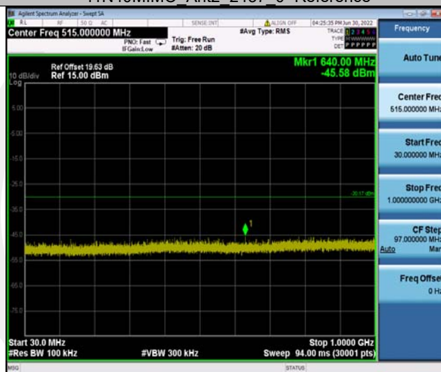
11N40MIMO_Ant2_2437_30~1000
