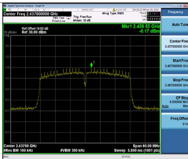
11N40MIMO_Ant2_2437_0~Reference
