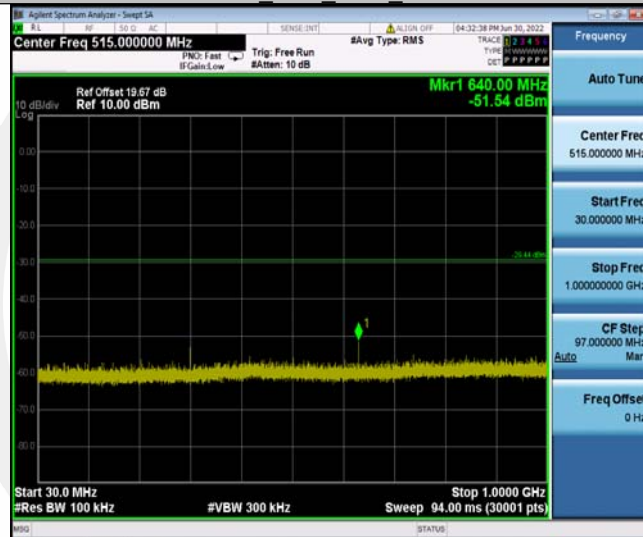
11N40MIMO_Ant1_2452_30~1000
