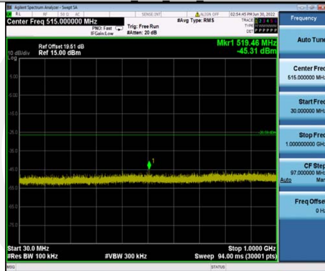
11N20MIMO_Ant1_2412_30~1000
