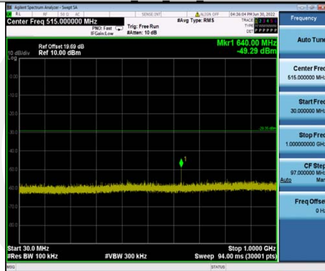
11N40MIMO_Ant2_2452_30~1000
