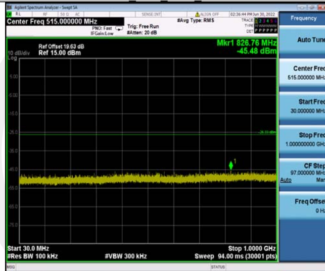
11N20SISO_Ant2_2437_30~1000
