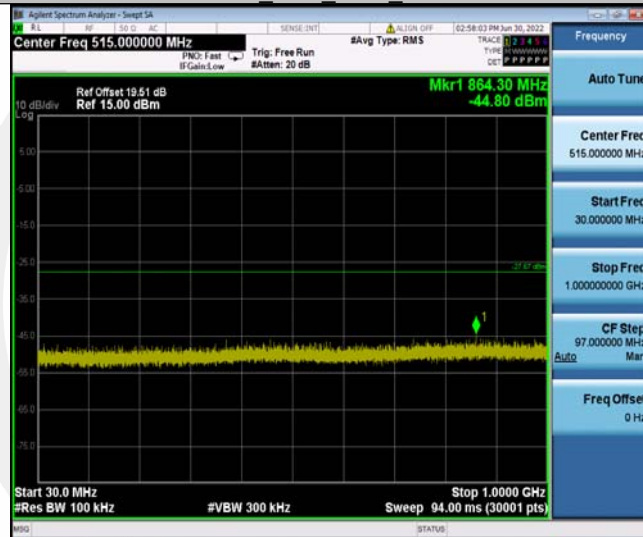
11N20MIMO_Ant2_2412_30~1000
