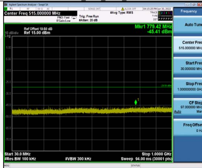
11N40MIMO_Ant1_2422_30~1000
