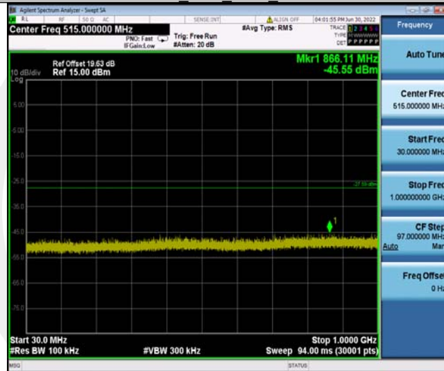
11N20MIMO_Ant2_2437_30~1000
