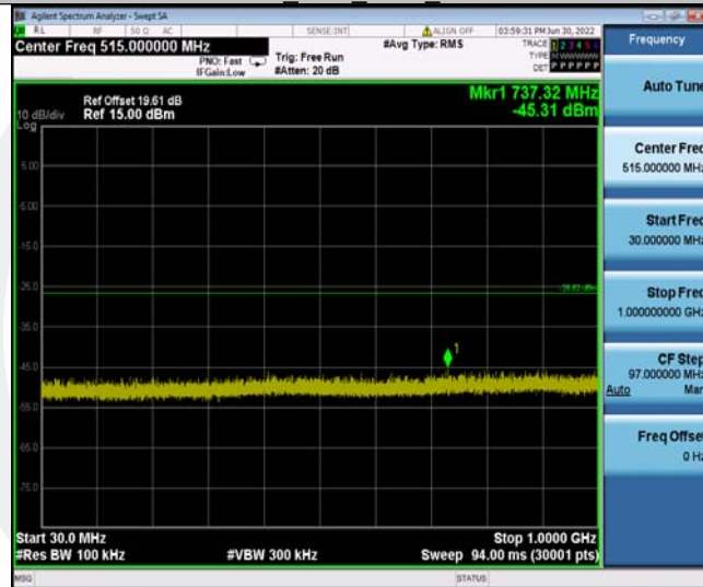
11N20MIMO_Ant1_2437_30~1000
