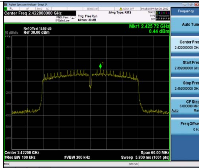
11N40MIMO_Ant1_2422_0~Reference
