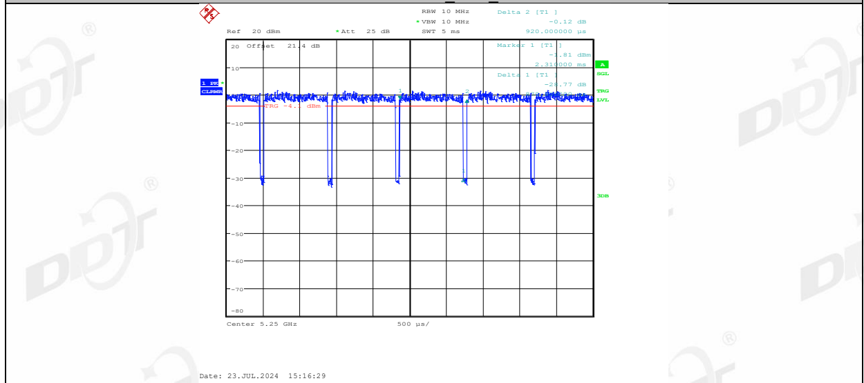
11AC160MIMO_Ant2_5250
