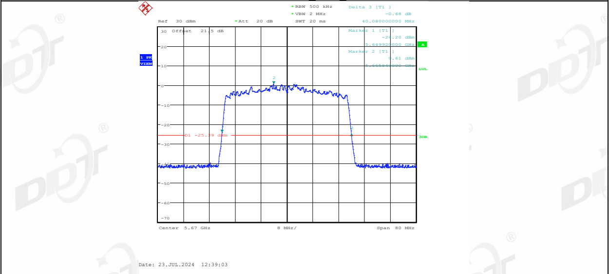
11AX40MIMO Ant2_5670
