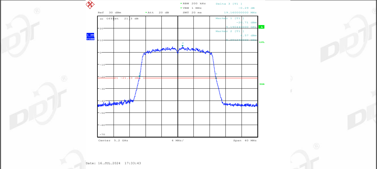
11N20MIMO_Ant2_5200
