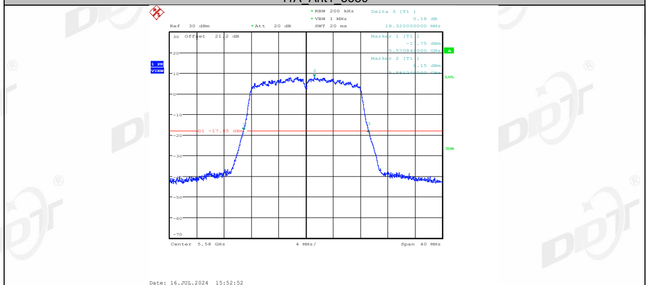
11A_Ant2_5580
