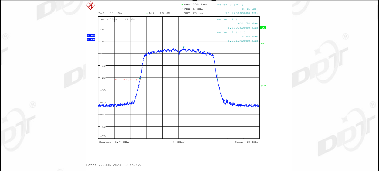
11AC20MIMO_Ant1_5720
