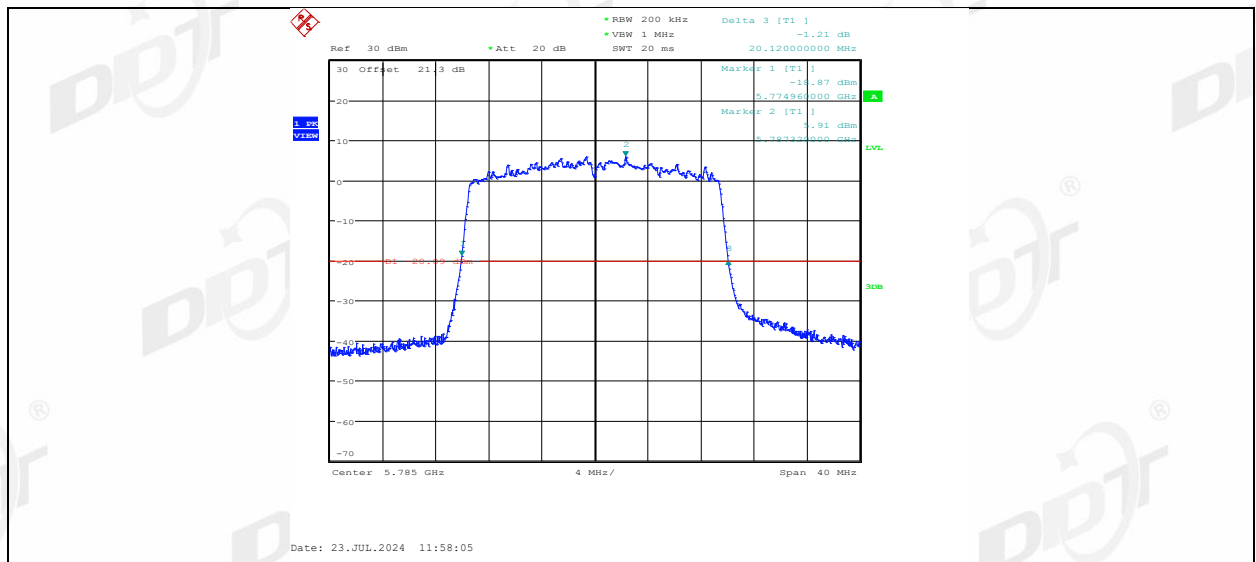
11AX20MIMO_Ant2_5785
