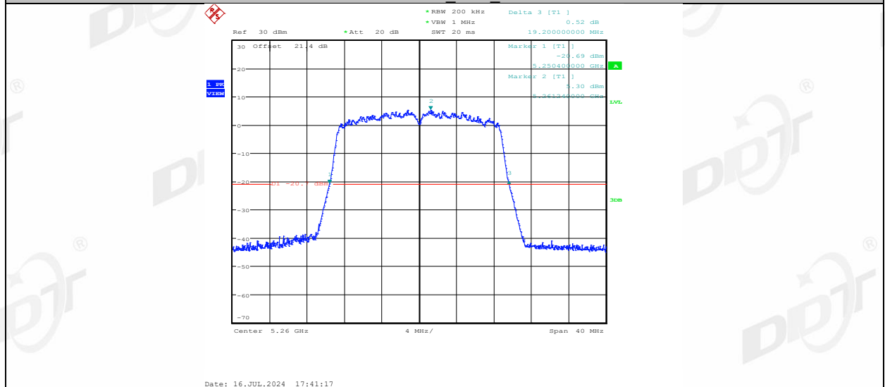
11N20MIMO_Ant2_5260
