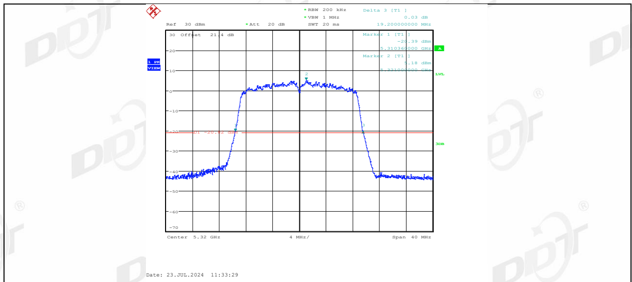
11AX20MIMO_Ant2_5320
