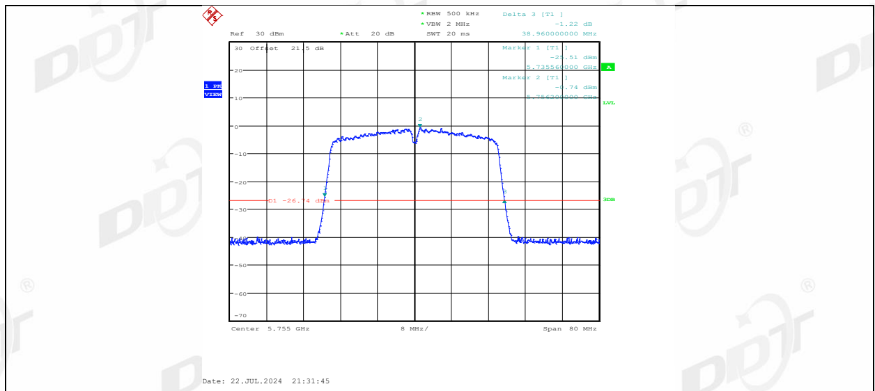
11AC40MIMO_Ant2_5755
