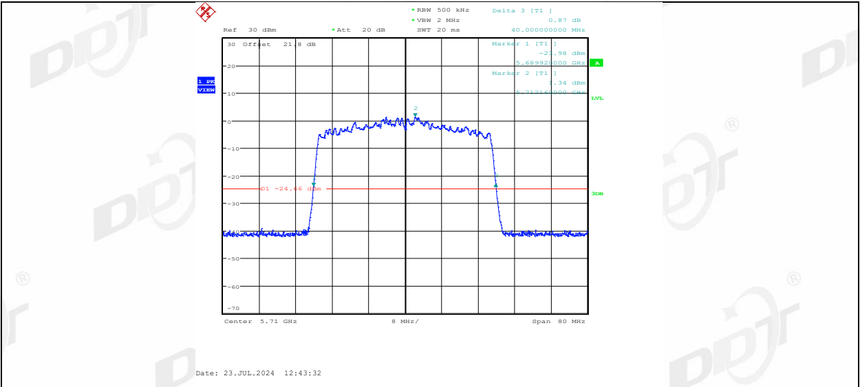
11AX40MIMO_Ant2_5710
