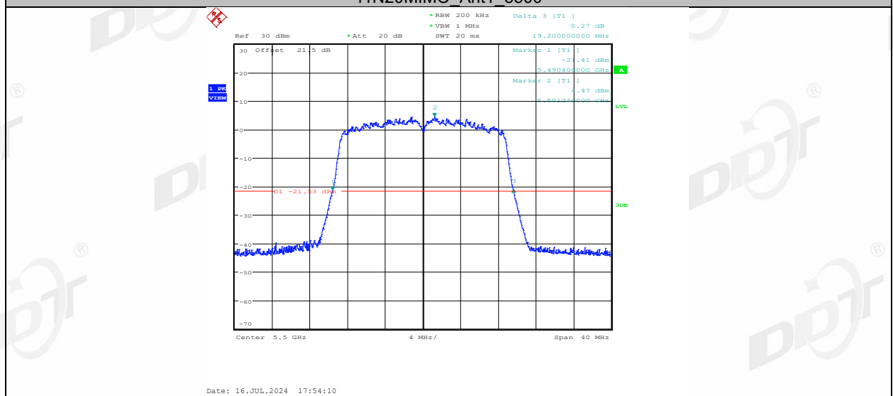
11N20MIMO Ant2 5500
