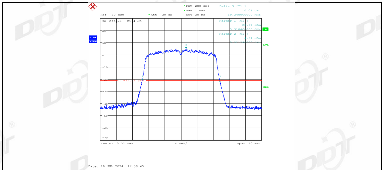
11N20MIMO_Ant2_5320
