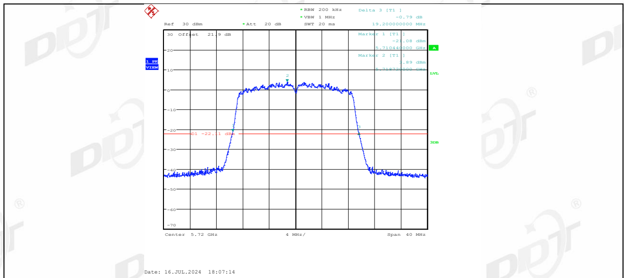
11N20MIMO_Ant1_5745
