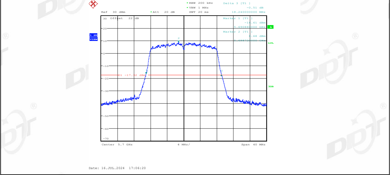
11A_Ant1_5720
