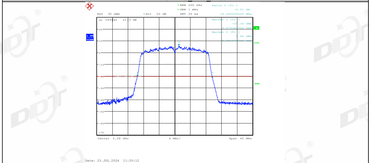
11AX20MIMO_Ant2_5280
