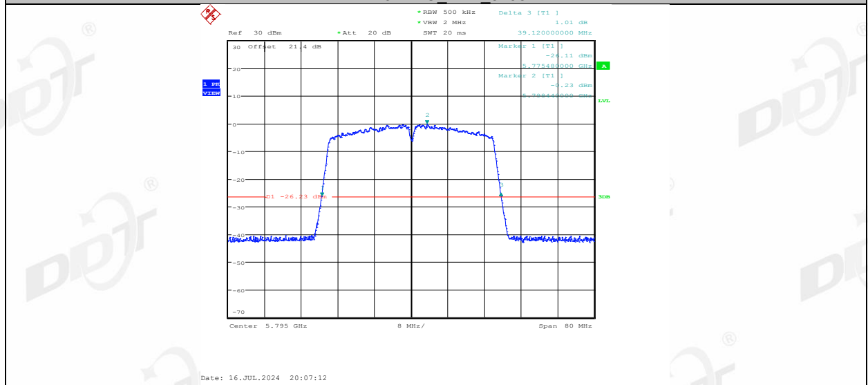
11N40MIMO_Ant2_5795
