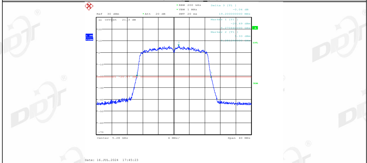
11N20MIMO_Ant2_5280
