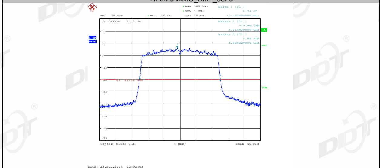
11AX20MIMO_Ant2_5825
