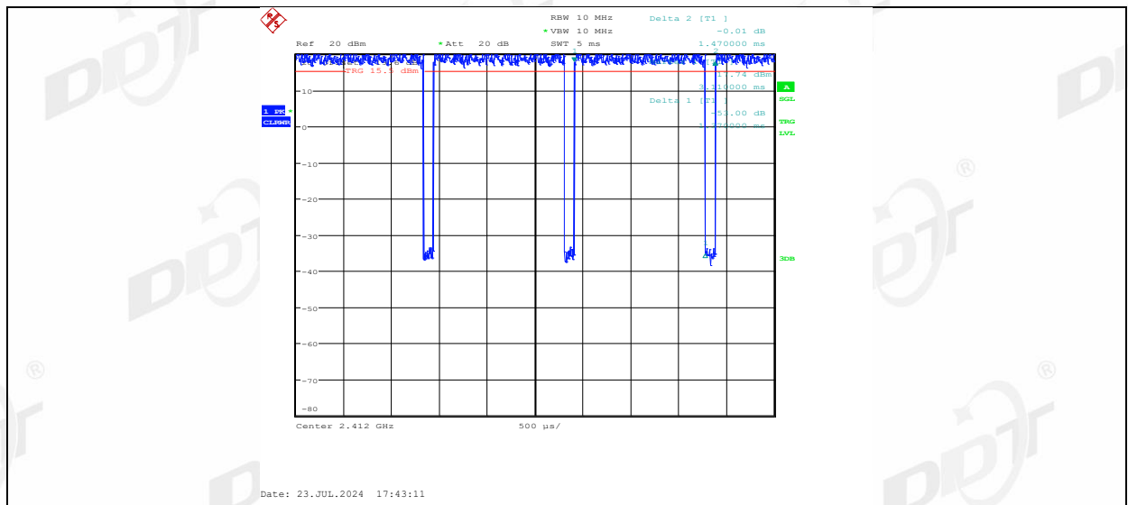
11G_Ant2_2412
