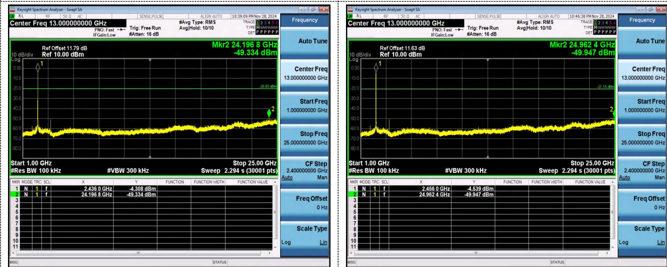
1GHz-25GHz
