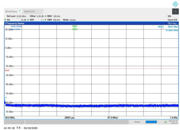
NTNV-n77(3700-3980)-PC3-30-90-L-DFT-QPSK-Edge_1RB_Left- 30-1000-PASS
