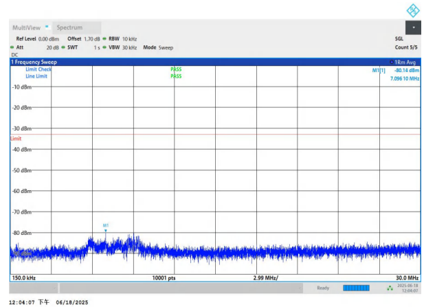
NTNV-n77(3700-3980)-PC3-30-90-L-DFT-BPSK-Edge_1RB_Left- 0.15-30-PASS
