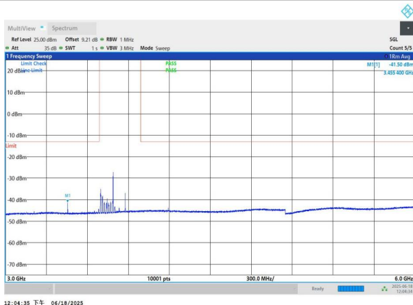
NTNV-n77(3700-3980)-PC3-30-90-L-DFT-BPSK-Edge_1RB_Left- 3000-6000-PASS
