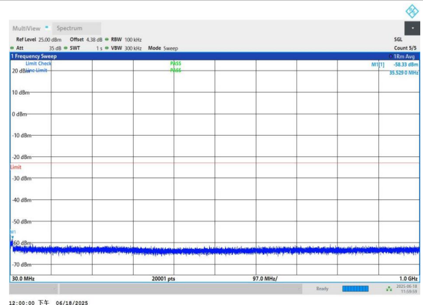
NTNV-n77(3700-3980)-PC3-30-80-M-DFT-QPSK-Edge_1RB_Left -30-1000-PASS
