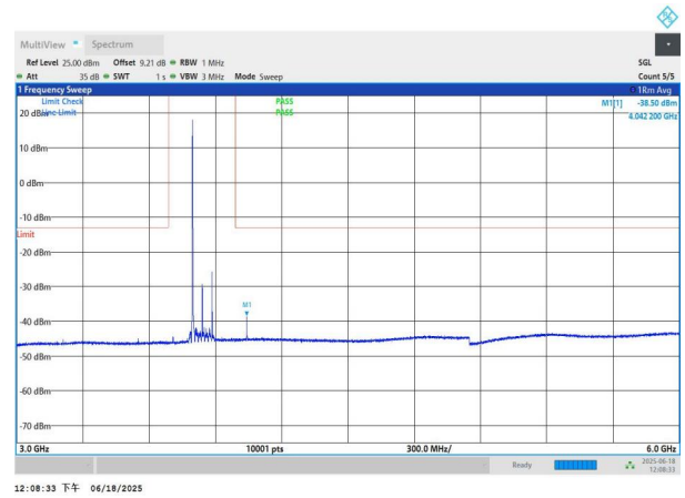
NTNV-n77(3700-3980)-PC3-30-90-M-DFT-QPSK-Edge_1RB_Left -3000-6000-PASS
