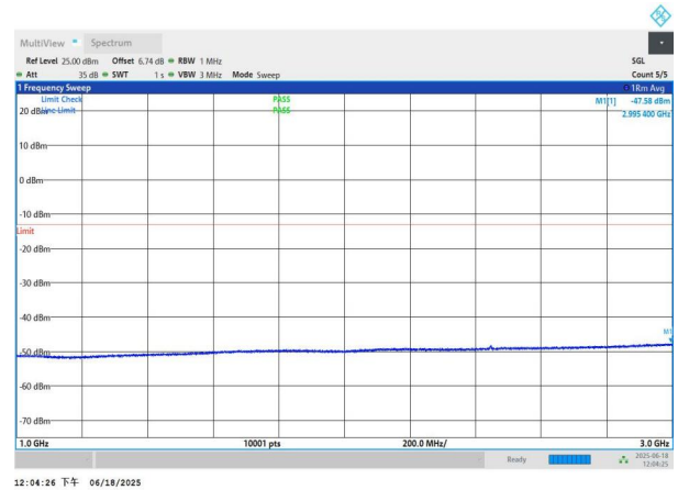
NTNV-n77(3700-3980)-PC3-30-90-L-DFT-BPSK-Edge_1RB_Left- 1000-3000-PASS
