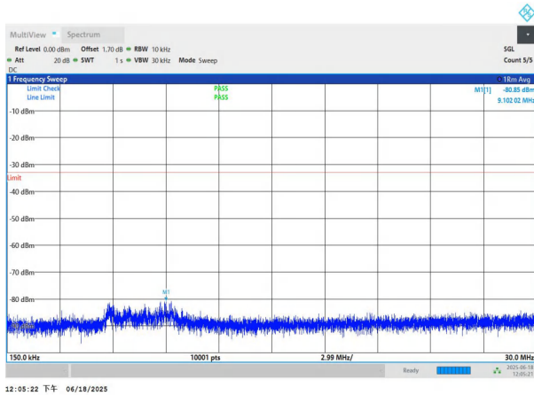
NTNV-n77(3700-3980)-PC3-30-90-L-DFT-QPSK-Edge_1RB_Left- 0.15-30-PASS
