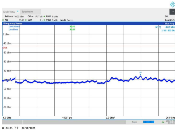
NTNV-n77(3700-3980)-PC3-30-90-L-DFT-QPSK-Edge_1RB_Left- 6000-26000-PASS
