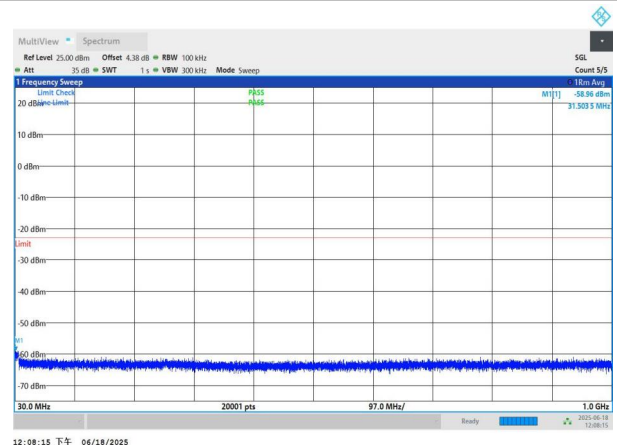
NTNV-n77(3700-3980)-PC3-30-90-M-DFT-QPSK-Edge_1RB_Left -30-1000-PASS
