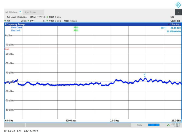
NTNV-n77(3700-3980)-PC3-30-90-L-DFT-BPSK-Edge_1RB_Left- 6000-26000-PASS
