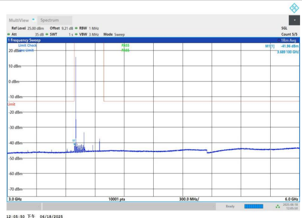
NTNV-n77(3700-3980)-PC3-30-90-L-DFT-QPSK-Edge_1RB_Left- 3000-6000-PASS
