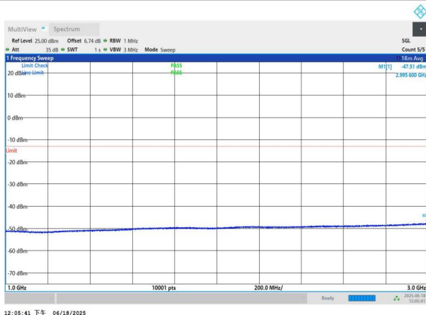
NTNV-n77(3700-3980)-PC3-30-90-L-DFT-QPSK-Edge_1RB_Left- 1000-3000-PASS
