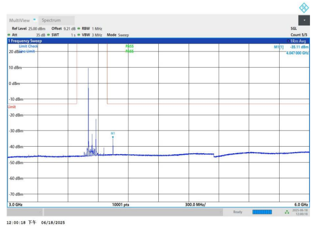
NTNV-n77(3700-3980)-PC3-30-80-M-DFT-QPSK-Edge_1RB_Left -3000-6000-PASS
