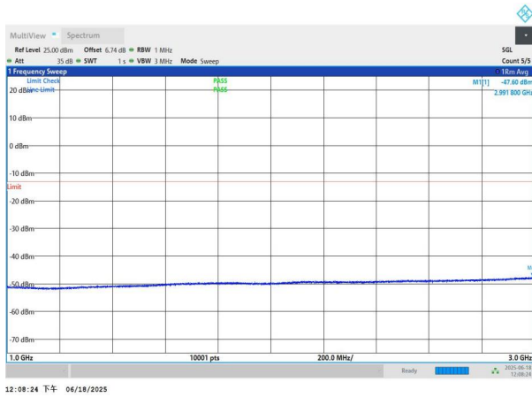
NTNV-n77(3700-3980)-PC3-30-90-M-DFT-QPSK-Edge_1RB_Left -1000-3000-PASS
