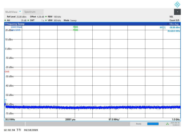
NTNV-n77(3700-3980)-PC3-30-80-H-DFT-QPSK-Edge_1RB_Left -30-1000-PASS
