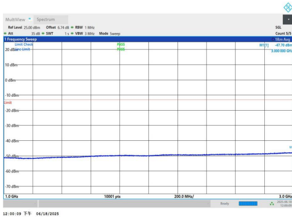
NTNV-n77(3700-3980)-PC3-30-80-M-DFT-QPSK-Edge_1RB_Left -1000-3000-PASS
