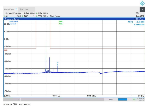
NTNV-n77(3700-3980)-PC3-30-80-H-DFT-QPSK-Edge_1RB_Left -3000-6000-PASS
