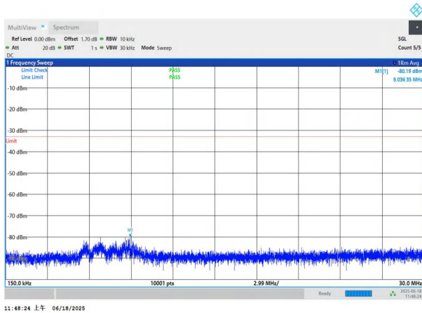
NTNV-n77(3700-3980)-PC3-30-70-L-DFT-QPSK-Edge_1RB_Left- 0.15-30-PASS
