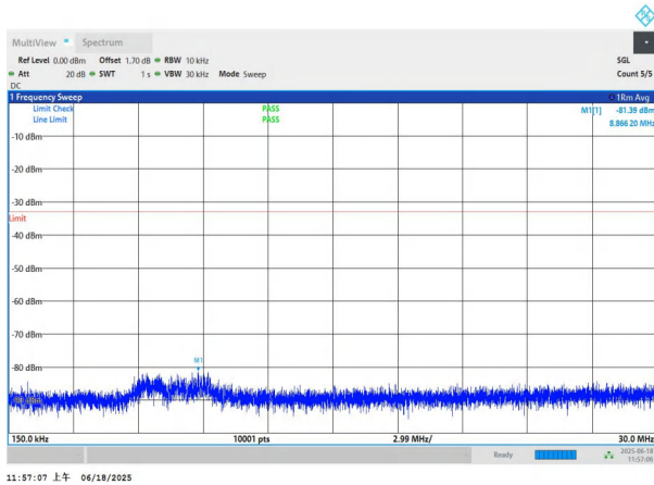
NTNV-n77(3700-3980)-PC3-30-80-L-DFT-QPSK-Edge_1RB_Left- 0.15-30-PASS
