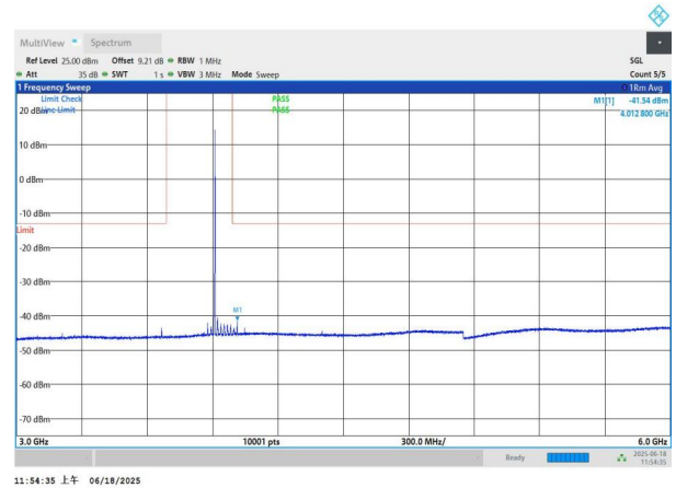
NTNV-n77(3700-3980)-PC3-30-70-H-DFT-QPSK-Edge_1RB_Left -3000-6000-PASS
