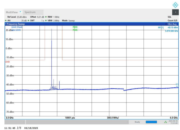
NTNV-n77(3700-3980)-PC3-30-70-M-DFT-QPSK-Edge_1RB_Left -3000-6000-PASS
