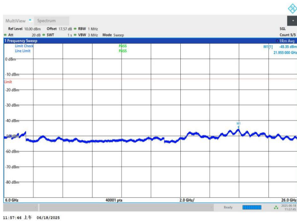
NTNV-n77(3700-3980)-PC3-30-80-L-DFT-QPSK-Edge_1RB_Left- 6000-26000-PASS
