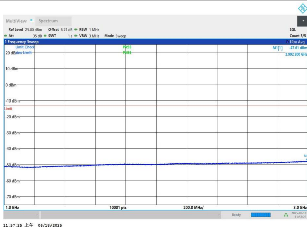
NTNV-n77(3700-3980)-PC3-30-80-L-DFT-QPSK-Edge_1RB_Left- 1000-3000-PASS
