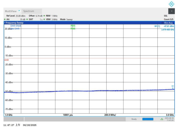
NTNV-n77(3700-3980)-PC3-30-70-L-DFT-BPSK-Edge_1RB_Left- 1000-3000-PASS
