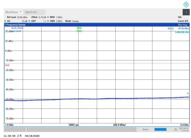
NTNV-n77(3700-3980)-PC3-30-80-L-DFT-BPSK-Edge_1RB_Left- 1000-3000-PASS
