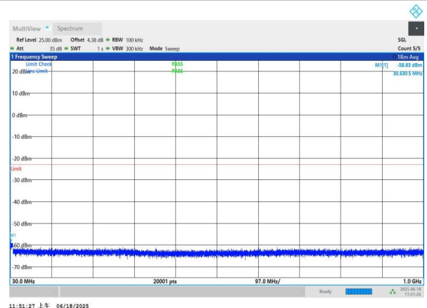
NTNV-n77(3700-3980)-PC3-30-70-M-DFT-QPSK-Edge_1RB_Left -30-1000-PASS
