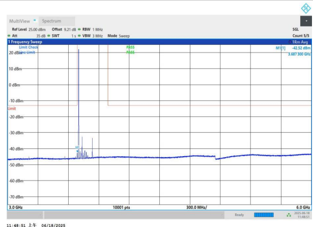
NTNV-n77(3700-3980)-PC3-30-70-L-DFT-QPSK-Edge_1RB_Left- 3000-6000-PASS
