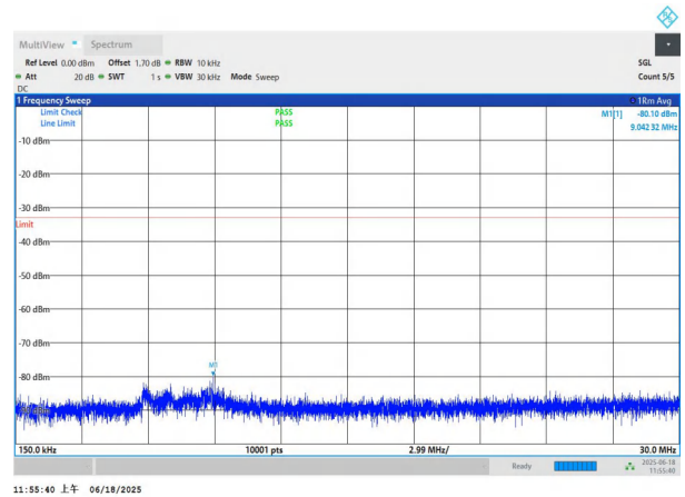
NTNV-n77(3700-3980)-PC3-30-80-L-DFT-BPSK-Edge_1RB_Left- 0.15-30-PASS
