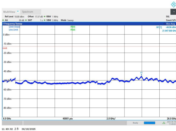
NTNV-n77(3700-3980)-PC3-30-70-L-DFT-QPSK-Edge_1RB_Left- 6000-26000-PASS
