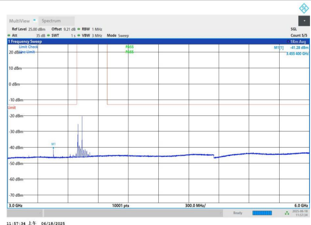
NTNV-n77(3700-3980)-PC3-30-80-L-DFT-QPSK-Edge_1RB_Left- 3000-6000-PASS
