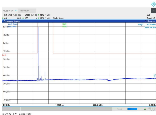
NTNV-n77(3700-3980)-PC3-30-70-L-DFT-BPSK-Edge_1RB_Left- 3000-6000-PASS
