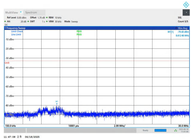
NTNV-n77(3700-3980)-PC3-30-70-L-DFT-BPSK-Edge_1RB_Left- 0.15-30-PASS
