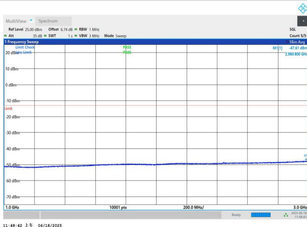
NTNV-n77(3700-3980)-PC3-30-70-L-DFT-QPSK-Edge_1RB_Left- 1000-3000-PASS
