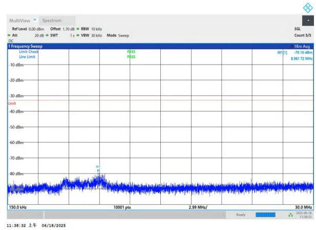
NTNV-n77(3700-3980)-PC3-30-60-L-DFT-BPSK-Edge_1RB_Left- 0.15-30-PASS
