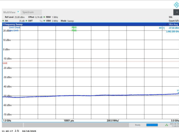
NTNV-n77(3700-3980)-PC3-30-60-L-DFT-QPSK-Edge_1RB_Left- 1000-3000-PASS
