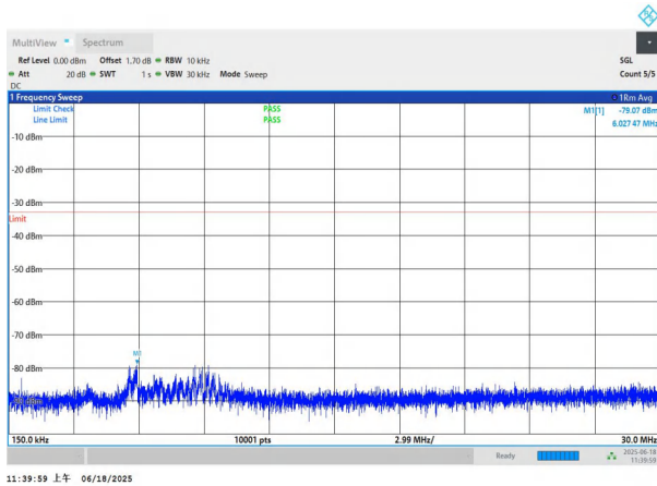
NTNV-n77(3700-3980)-PC3-30-60-L-DFT-QPSK-Edge_1RB_Left- 0.15-30-PASS
