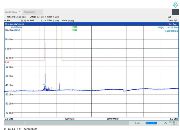
NTNV-n77(3700-3980)-PC3-30-60-L-DFT-QPSK-Edge_1RB_Left- 3000-6000-PASS
