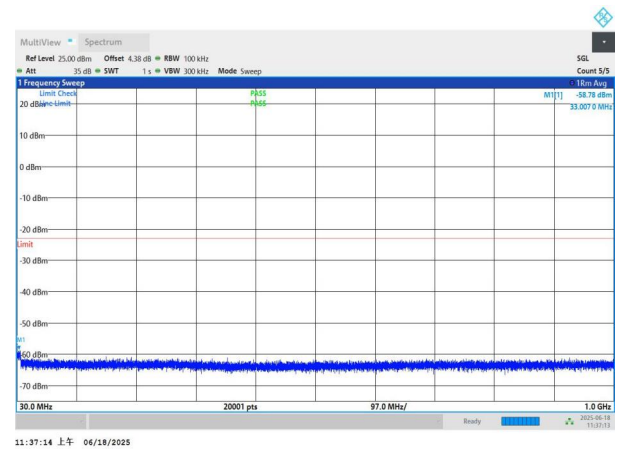
NTNV-n77(3700-3980)-PC3-30-50-H-DFT-QPSK-Edge_1RB_Left -30-1000-PASS
