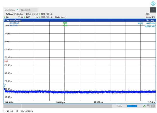
NTNV-n77(3700-3980)-PC3-30-60-L-DFT-QPSK-Edge_1RB_Left- 30-1000-PASS
