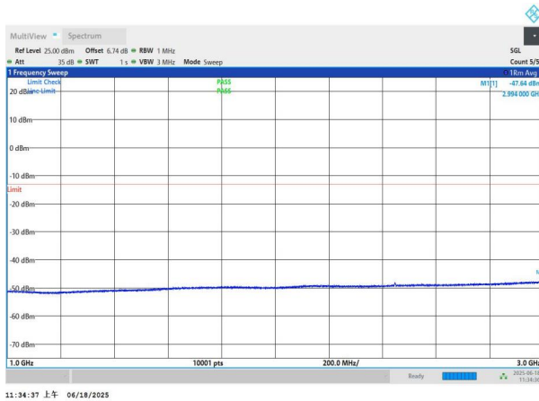
NTNV-n77(3700-3980)-PC3-30-50-M-DFT-QPSK-Edge_1RB_Left -1000-3000-PASS
