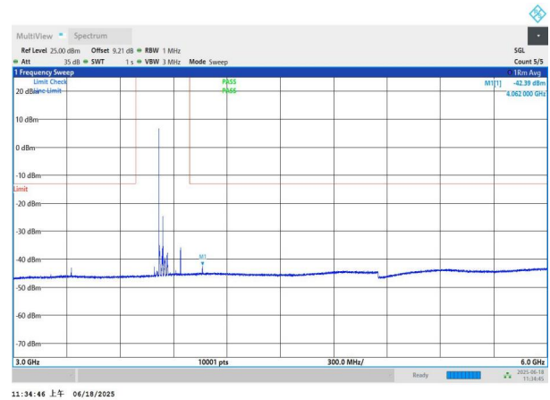
NTNV-n77(3700-3980)-PC3-30-50-M-DFT-QPSK-Edge_1RB_Left -3000-6000-PASS
