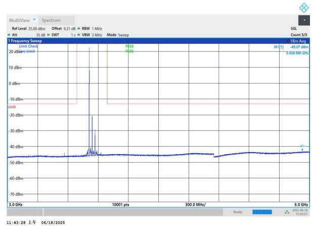
NTNV-n77(3700-3980)-PC3-30-60-M-DFT-QPSK-Edge_1RB_Left -3000-6000-PASS
