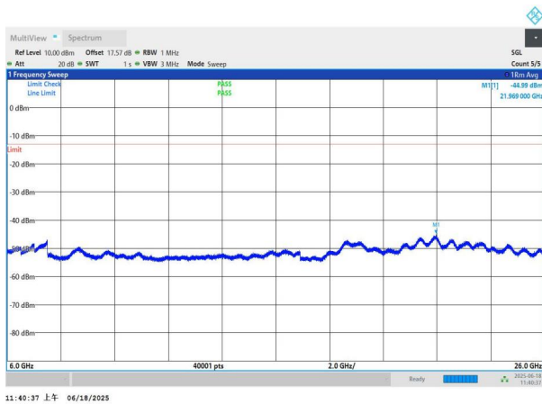
NTNV-n77(3700-3980)-PC3-30-60-L-DFT-QPSK-Edge_1RB_Left- 6000-26000-PASS
