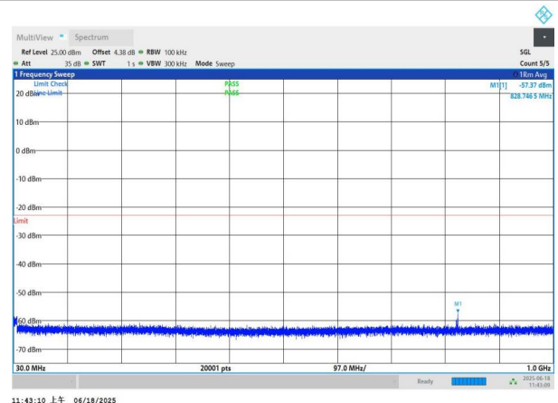
NTNV-n77(3700-3980)-PC3-30-60-M-DFT-QPSK-Edge_1RB_Left -30-1000-PASS
