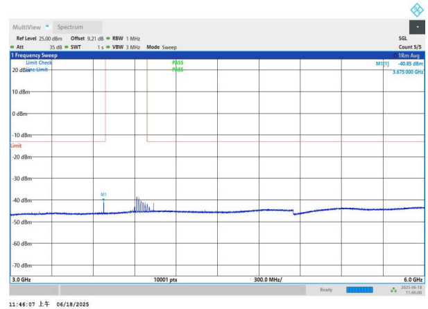
NTNV-n77(3700-3980)-PC3-30-60-H-DFT-QPSK-Edge_1RB_Left -3000-6000-PASS
