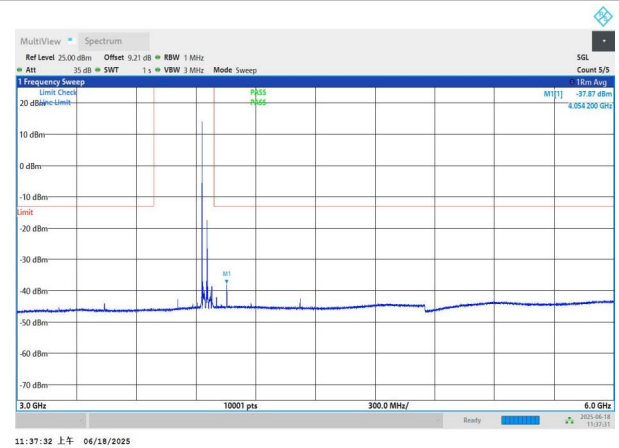
NTNV-n77(3700-3980)-PC3-30-50-H-DFT-QPSK-Edge_1RB_Left -3000-6000-PASS
