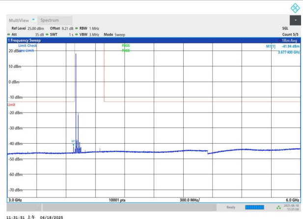
NTNV-n77(3700-3980)-PC3-30-50-L-DFT-QPSK-Edge_1RB_Left- 3000-6000-PASS
