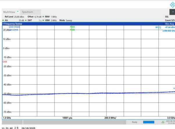
NTNV-n77(3700-3980)-PC3-30-50-L-DFT-QPSK-Edge_1RB_Left- 1000-3000-PASS
