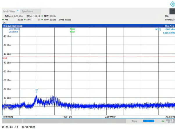
NTNV-n77(3700-3980)-PC3-30-50-L-DFT-QPSK-Edge_1RB_Left- 0.15-30-PASS
