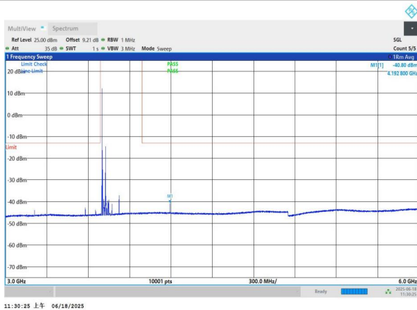
NTNV-n77(3700-3980)-PC3-30-50-L-DFT-BPSK-Edge_1RB_Left- 3000-6000-PASS
