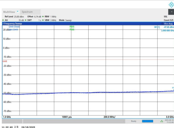
NTNV-n77(3700-3980)-PC3-30-40-L-DFT-QPSK-Edge_1RB_Left- 1000-3000-PASS
