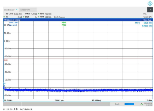
NTNV-n77(3700-3980)-PC3-30-40-L-DFT-QPSK-Edge_1RB_Left- 30-1000-PASS
