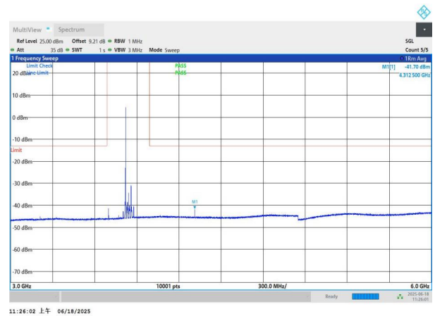
NTNV-n77(3700-3980)-PC3-30-40-M-DFT-QPSK-Edge_1RB_Left -3000-6000-PASS
