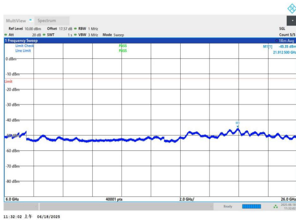
NTNV-n77(3700-3980)-PC3-30-50-L-DFT-QPSK-Edge_1RB_Left- 6000-26000-PASS
