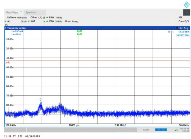
NTNV-n77(3700-3980)-PC3-30-50-L-DFT-BPSK-Edge_1RB_Left- 0.15-30-PASS
