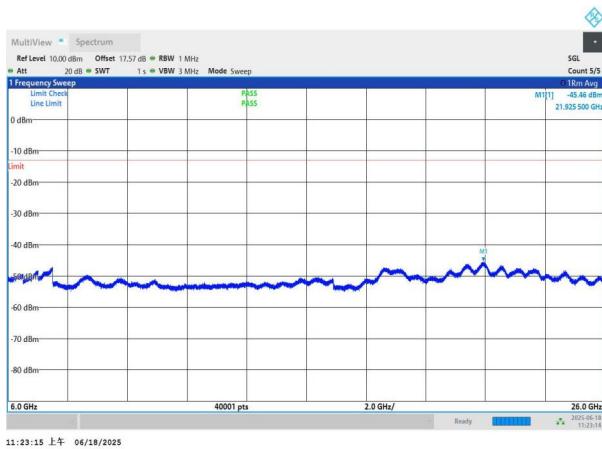
NTNV-n77(3700-3980)-PC3-30-40-L-DFT-QPSK-Edge_1RB_Left- 6000-26000-PASS
