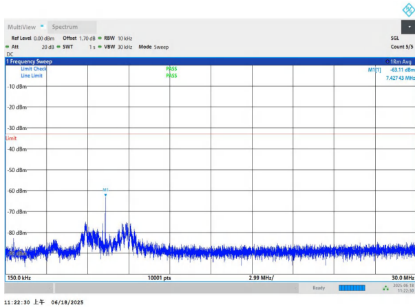
NTNV-n77(3700-3980)-PC3-30-40-L-DFT-QPSK-Edge_1RB_Left- 0.15-30-PASS
