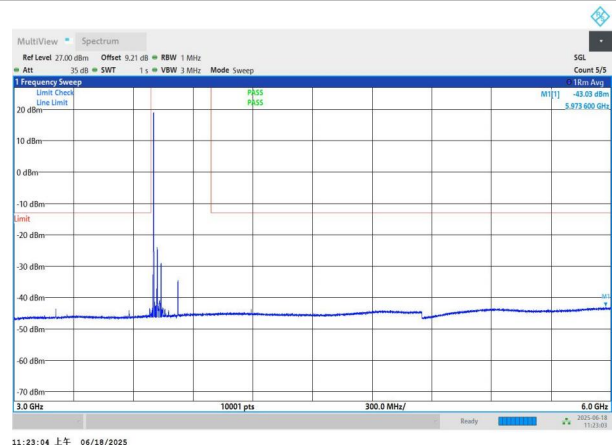
NTNV-n77(3700-3980)-PC3-30-40-L-DFT-QPSK-Edge_1RB_Left- 3000-6000-PASS
