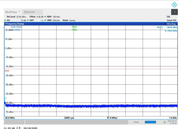
NTNV-n77(3700-3980)-PC3-30-40-M-DFT-QPSK-Edge_1RB_Left -30-1000-PASS
