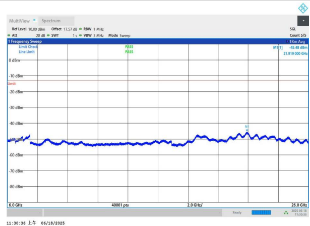
NTNV-n77(3700-3980)-PC3-30-50-L-DFT-BPSK-Edge_1RB_Left- 6000-26000-PASS
