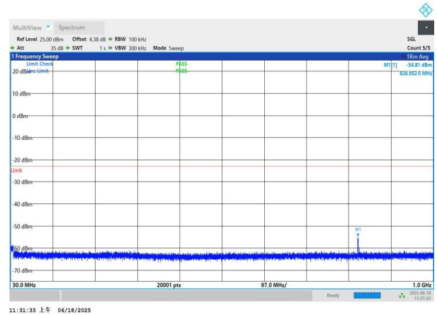
NTNV-n77(3700-3980)-PC3-30-50-L-DFT-QPSK-Edge_1RB_Left- 30-1000-PASS
