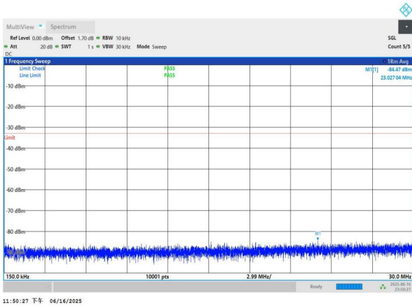
NTNV-n77(3450-3550)-PC3-30-90-L-DFT-QPSK-Edge_1RB_Left- 0.15-30-PASS
