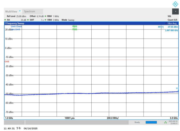
NTNV-n77(3450-3550)-PC3-30-90-L-DFT-BPSK-Edge_1RB_Left-30-1000-PASS NTVN-n77(3450-3550)-PC3-30-90-L-DFT-BPSK-Edge_1RB_Left-1000-3000-PASS
