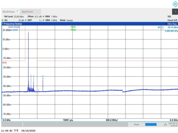
NTNV-n77(3450-3550)-PC3-30-90-L-DFT-BPSK-Edge_1RB_Left-3000-6000-PASS NTVN-n77(3450-3550)-PC3-30-90-L-DFT-BPSK-Edge_1RB_Left-6000-20000-PASS
