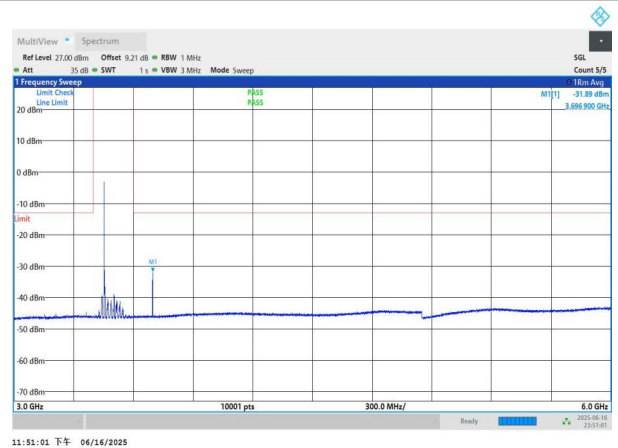
NTNV-n77(3450-3550)-PC3-30-90-L-DFT-QPSK-Edge_1RB_Left- 3000-6000-PASS
