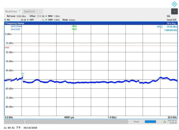
NTNV-n77(3450-3550)-PC3-30-90-L-DFT-BPSK-Edge_1RB_Left-3000-6000-PASS NTVN-n77(3450-3550)-PC3-30-90-L-DFT-BPSK-Edge_1RB_Left-6000-20000-PASS
