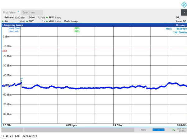
NTNV-n77(3450-3550)-PC3-30-80-L-DFT-QPSK-Edge_1RB_Left-6000-20000-PASS
