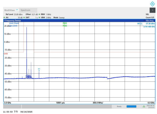
NTNV-n77(3450-3550)-PC3-30-90-M-DFT-QPSK-Edge_1RB_Left -3000-6000-PASS
