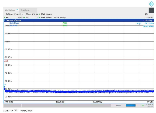
NTNV-n77(3450-3550)-PC3-30-80-H-DFT-QPSK-Edge_1RB_Left -30-1000-PASS
