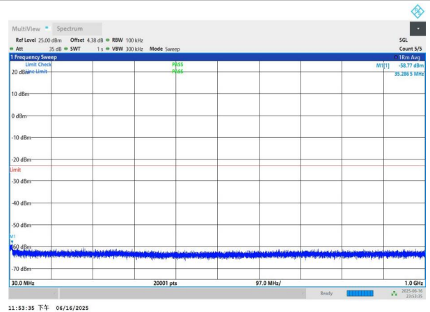
NTNV-n77(3450-3550)-PC3-30-90-M-DFT-QPSK-Edge_1RB_Left -30-1000-PASS
