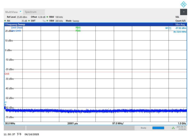
NTNV-n77(3450-3550)-PC3-30-90-L-DFT-QPSK-Edge_1RB_Left- 30-1000-PASS
