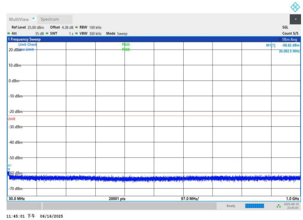
NTNV-n77(3450-3550)-PC3-30-80-M-DFT-QPSK-Edge_1RB_Left -30-1000-PASS
