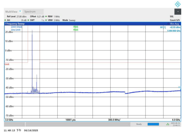
NTNV-n77(3450-3550)-PC3-30-80-H-DFT-QPSK-Edge_1RB_Left -3000-6000-PASS
