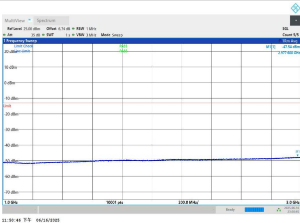
NTNV-n77(3450-3550)-PC3-30-90-L-DFT-QPSK-Edge_1RB_Left- 1000-3000-PASS
