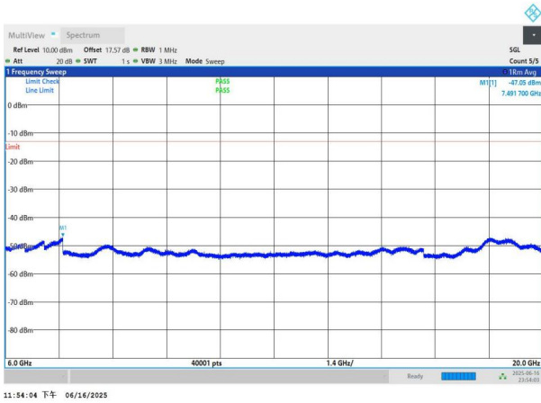
NTNV-n77(3450-3550)-PC3-30-90-M-DFT-QPSK-Edge_1RB_Left -6000-20000-PASS
