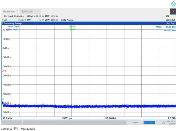
NTNV-n77(3450-3550)-PC3-30-90-M-DFT-BPSK-Edge_1RB_Left-30-1000-PASS
