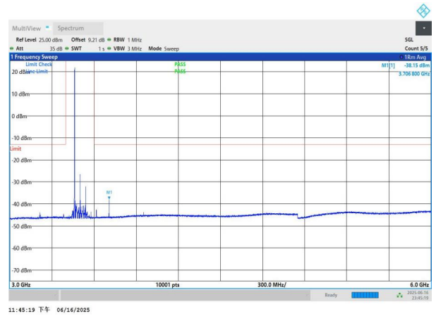
NTNV-n77(3450-3550)-PC3-30-80-M-DFT-QPSK-Edge_1RB_Left -3000-6000-PASS
