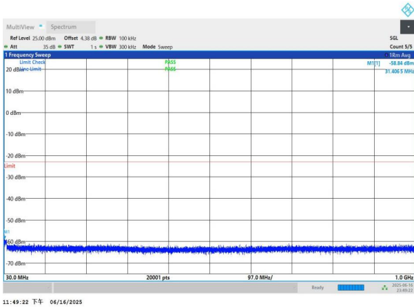
NTNV-n77(3450-3550)-PC3-30-90-L-DFT-BPSK-Edge_1RB_Left-30-1000-PASS NTVN-n77(3450-3550)-PC3-30-90-L-DFT-BPSK-Edge_1RB_Left-1000-3000-PASS
