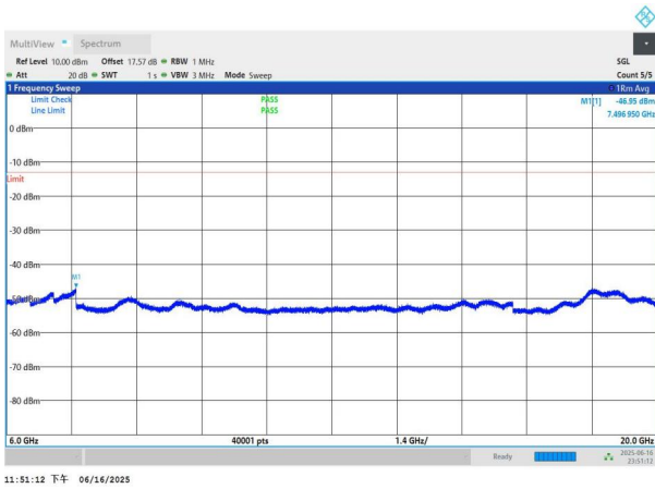
NTNV-n77(3450-3550)-PC3-30-90-L-DFT-QPSK-Edge_1RB_Left-6000-20000-PASS
