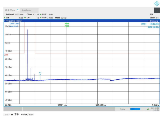
NTNV-n77(3450-3550)-PC3-30-70-L-DFT-QPSK-Edge_1RB_Left- 3000-6000-PASS
