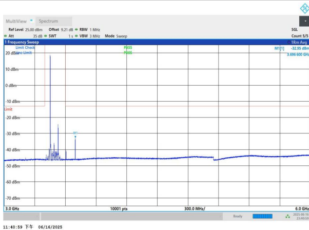
NTNV-n77(3450-3550)-PC3-30-80-L-DFT-BPSK-Edge_1RB_Left- 3000-6000-PASS
