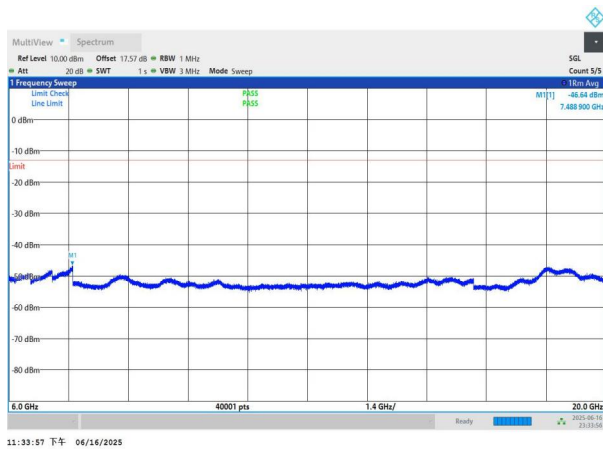
NTNV-n77(3450-3550)-PC3-30-70-L-DFT-QPSK-Edge_1RB_Left- 6000-20000-PASS
