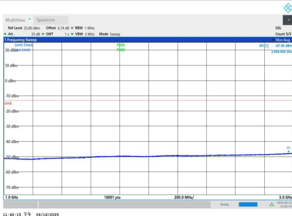
NTNV-n77(3450-3550)-PC3-30-80-L-DFT-QPSK-Edge_1RB_Left- 1000-3000-PASS
