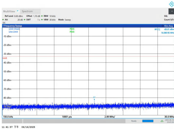
NTNV-n77(3450-3550)-PC3-30-80-L-DFT-QPSK-Edge_1RB_Left- 0.15-30-PASS
