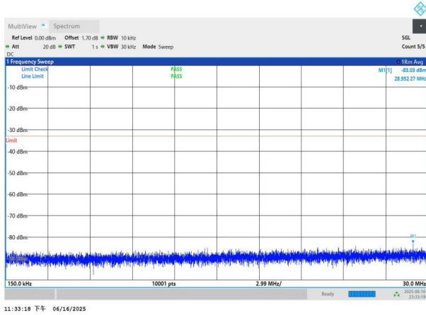
NTNV-n77(3450-3550)-PC3-30-70-L-DFT-QPSK-Edge_1RB_Left- 0.15-30-PASS
