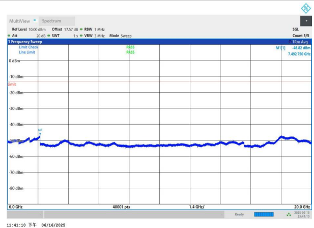
NTNV-n77(3450-3550)-PC3-30-80-L-DFT-BPSK-Edge_1RB_Left- 6000-20000-PASS
