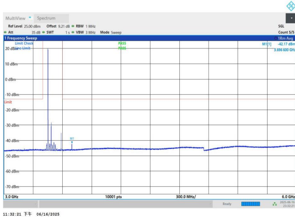
NTNV-n77(3450-3550)-PC3-30-70-L-DFT-BPSK-Edge_1RB_Left- 3000-6000-PASS
