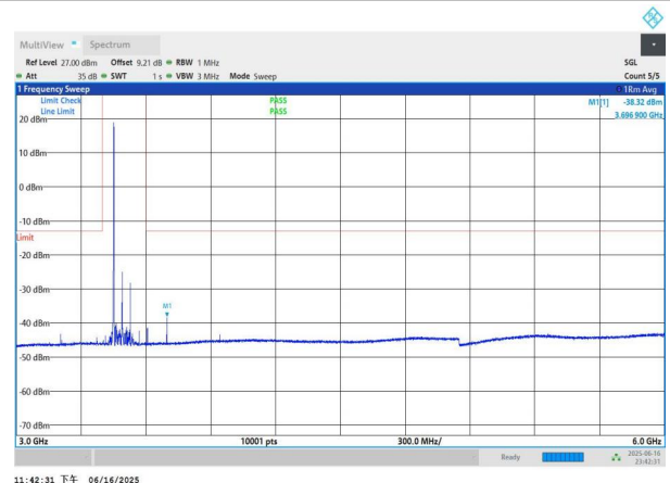
NTNV-n77(3450-3550)-PC3-30-80-L-DFT-QPSK-Edge_1RB_Left- 3000-6000-PASS
