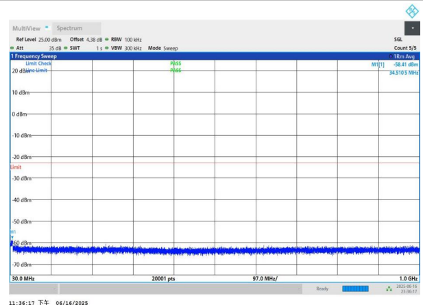
NTNV-n77(3450-3550)-PC3-30-70-M-DFT-QPSK-Edge_1RB_Left -30-1000-PASS
