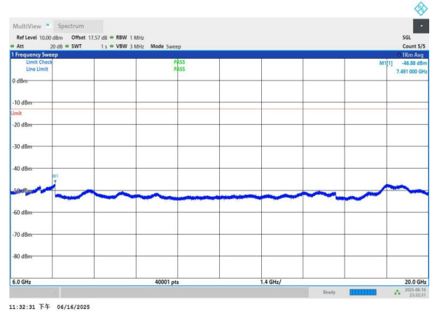
NTNV-n77(3450-3550)-PC3-30-70-L-DFT-BPSK-Edge_1RB_Left- 6000-20000-PASS
