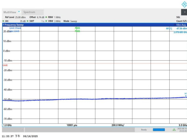
NTNV-n77(3450-3550)-PC3-30-70-L-DFT-QPSK-Edge_1RB_Left- 1000-3000-PASS
