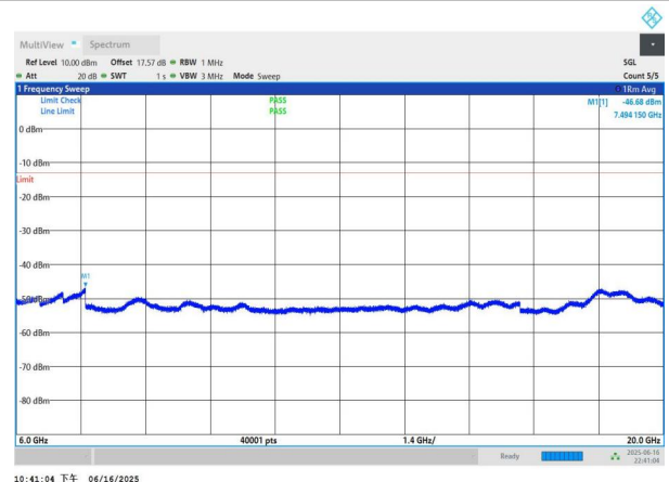
NTNV-n77(3450-3550)-PC3-30-20-L-DFT-BPSK-Edge_1RB_Left- 6000-20000-PASS
