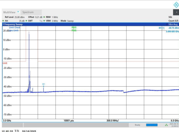
NTNV-n77(3450-3550)-PC3-30-20-L-DFT-BPSK-Edge_1RB_Left- 3000-6000-PASS
