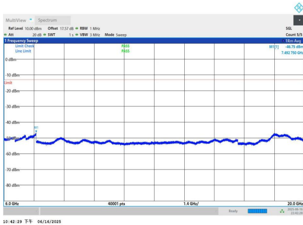
NTNV-n77(3450-3550)-PC3-30-20-L-DFT-QPSK-Edge_1RB_Left- 6000-20000-PASS
