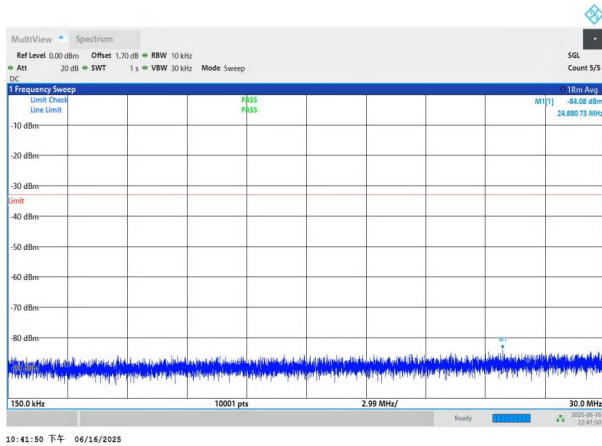
NTNV-n77(3450-3550)-PC3-30-20-L-DFT-QPSK-Edge_1RB_Left- 0.15-30-PASS
