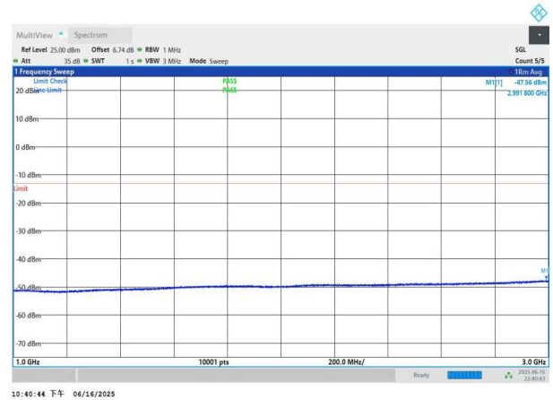
NTNV-n77(3450-3550)-PC3-30-20-L-DFT-BPSK-Edge_1RB_Left- 1000-3000-PASS
