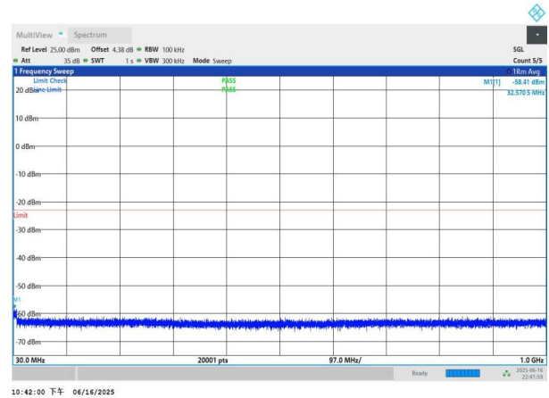
NTNV-n77(3450-3550)-PC3-30-20-L-DFT-QPSK-Edge_1RB_Left- 30-1000-PASS
