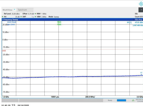
NTNV-n77(3450-3550)-PC3-30-20-L-DFT-QPSK-Edge_1RB_Left- 1000-3000-PASS
