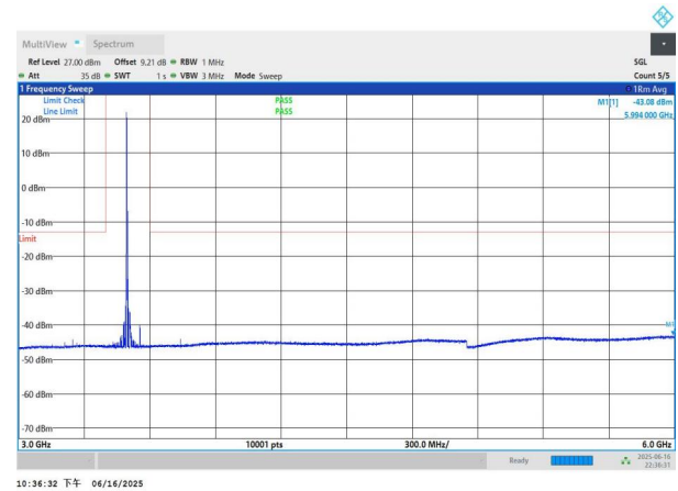
NTNV-n77(3450-3550)-PC3-30-15-M-DFT-QPSK-Edge_1RB_Left -3000-6000-PASS
