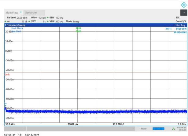
NTNV-n77(3450-3550)-PC3-30-15-M-DFT-QPSK-Edge_1RB_Left -30-1000-PASS
