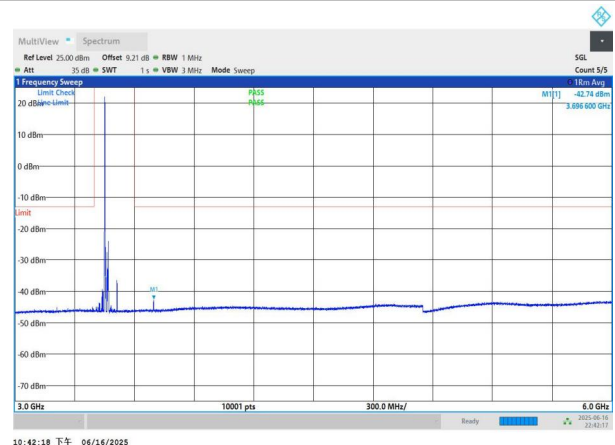
NTNV-n77(3450-3550)-PC3-30-20-L-DFT-QPSK-Edge_1RB_Left- 3000-6000-PASS
