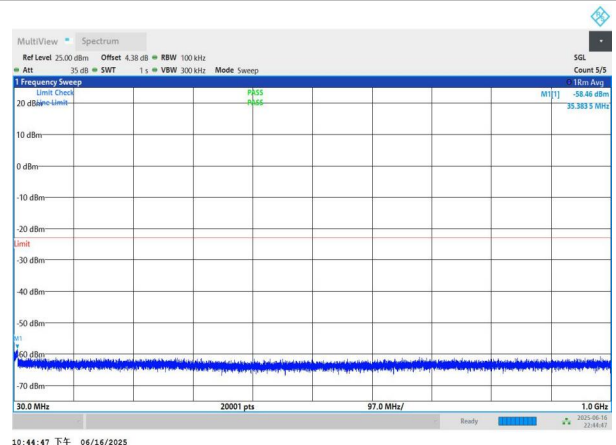
NTNV-n77(3450-3550)-PC3-30-20-M-DFT-QPSK-Edge_1RB_Left -30-1000-PASS
