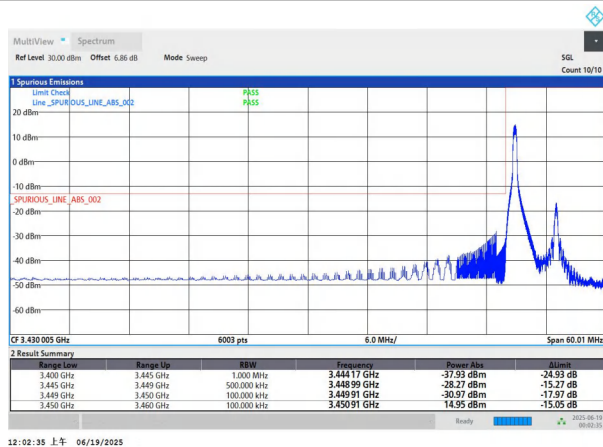
NTNV-n77(3450-3550)-PC3-30-10-L-DFT-QPSK-Edge_1RB_Left-PA SS
