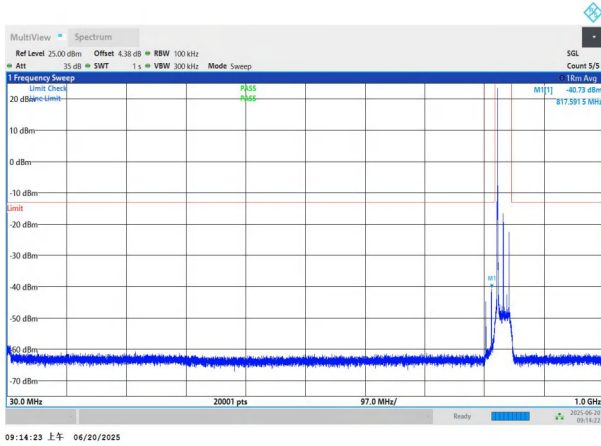
NTNV-n26(824-849)-PC3-15-20-M-DFT-QPSK-Edge_1RB_Left-3.0-1000-PASS
