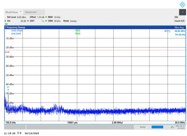
NTNV-n26(824-849)-PC3-15-10-M-DFT-QPSK-Edge_1RB_Left-0. 15-30-PASS
