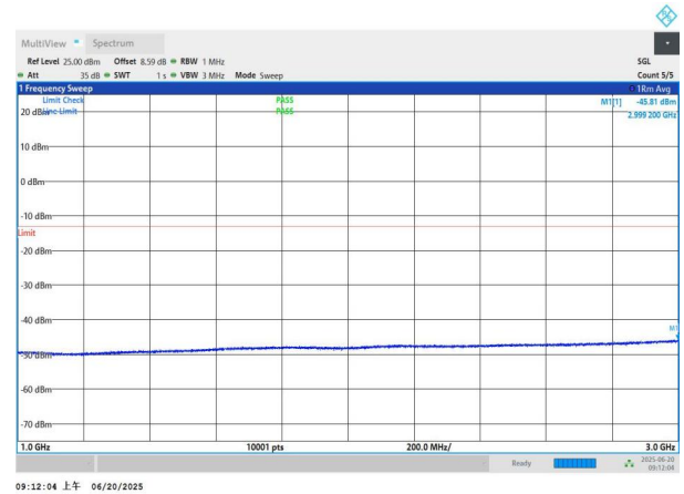
NTNV-n26(824-849)-PC3-15-20-L-DFT-QPSK-Edge_1RB_Left-10 00-3000-PASS
