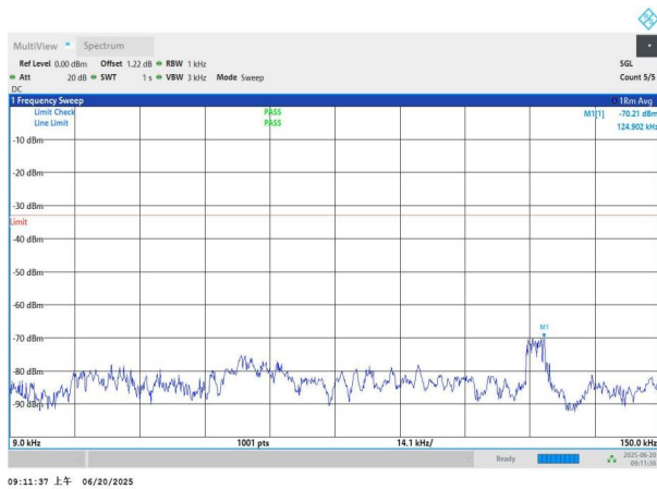
NTNV-n26(824-849)-PC3-15-20-L-DFT-QPSK-Edge_1RB_Left-0. 009-0.15-PASS
