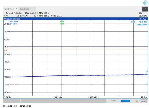
NTNV-n26(824-849)-PC3-15-20-M-DFT-QPSK-Edge_1RB_Left-10.00-3000-PASS
