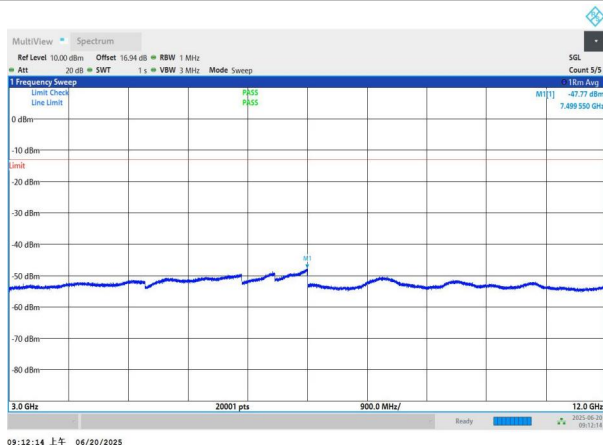
NTNV-n26(824-849)-PC3-15-20-L-DFT-QPSK-Edge_1RB_Left-3 000-12000-PASS
