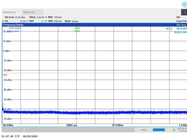
NTNV-n66-PC3-15-20-M-DFT-BPSK-Edge_1RB_Left-30-1000-P ASS
