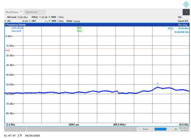
NTNV-n66-PC3-15-20-M-DFT-BPSK-Edge_1RB_Left-12000-2000 0-PASS
