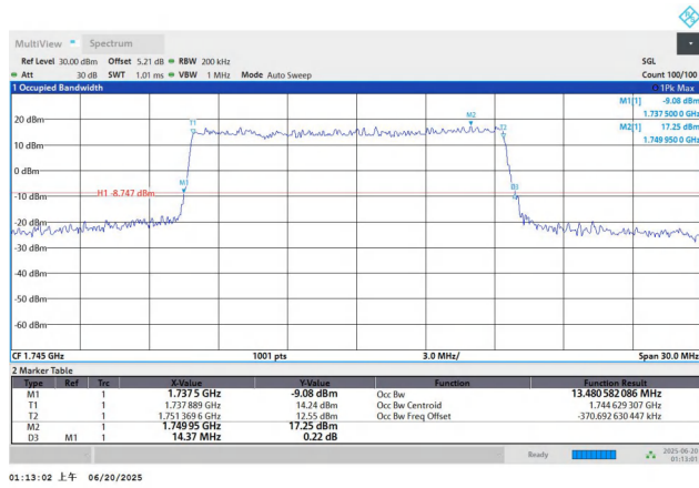
NTNV-n66-PC3-15-15-M-DFT-QPSK-Outet_Full-Ant1-PASS
