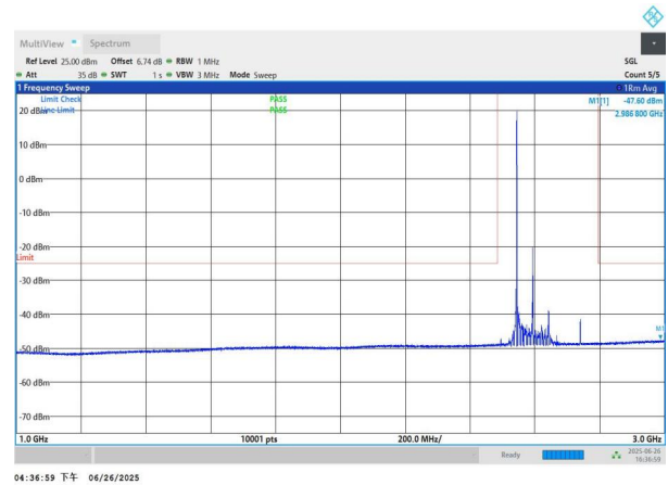
NTNV-n41-PC3-30-100-M-DFT-QPSK-Edge_1RB_Left-1000-3000- -PASS
