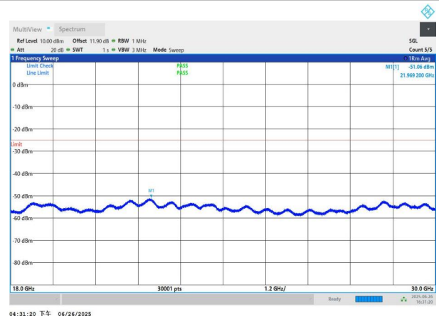
NTNV-n41-PC3-30-90-M-DFT-BPSK-Edge_1RB_Left-18000-3000 0-PASS
