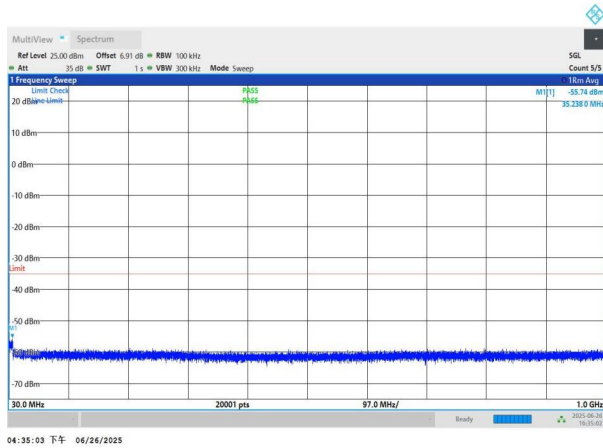
NTNV-n41-PC3-30-100-L-DFT-QPSK-Edge_1RB_Left-30-1000-P ASS
