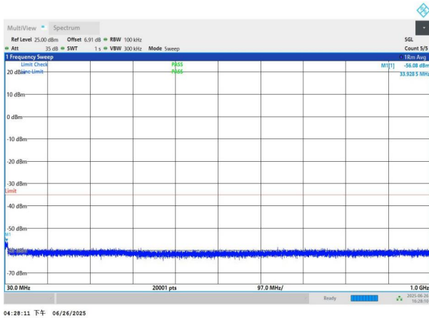
NTNV-n41-PC3-30-80-H-DFT-QPSK-Edge_1RB_Left-30-1000-P ASS
