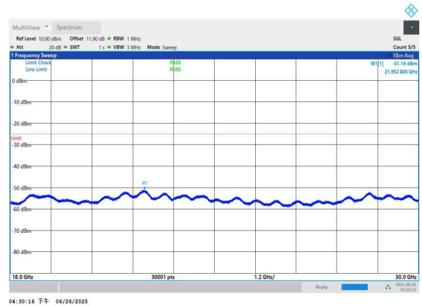
NTNV-n41-PC3-30-90-L-DFT-QPSK-Edge_1RB_Left-18000-3000 0-PASS
