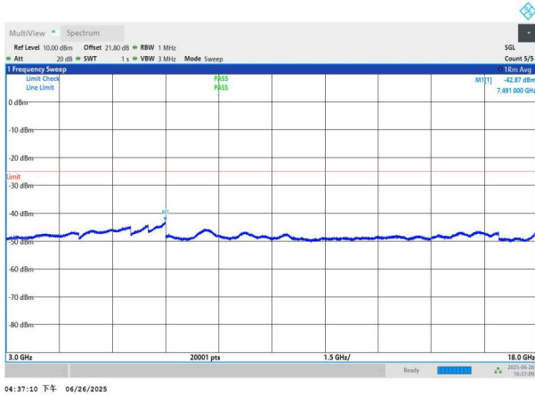
NTNV-n41-PC3-30-100-M-DFT-QPSK-Edge_1RB_Left-3000-180 00-PASS
