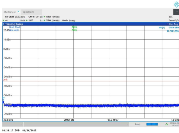
NTNV-n41-PC3-30-100-L-DFT-BPSK-Edge_1RB_Left-30-1000-P ASS
