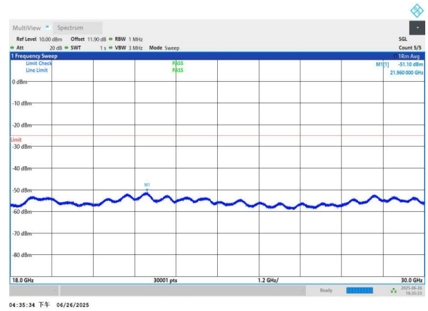
NTNV-n41-PC3-30-100-L-DFT-QPSK-Edge_1RB_Left-18000-300 00-PASS
