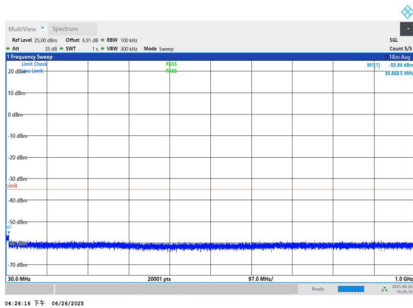
NTNV-n41-PC3-30-80-M-DFT-QPSK-Edge_1RB_Left-30-1000-P ASS
