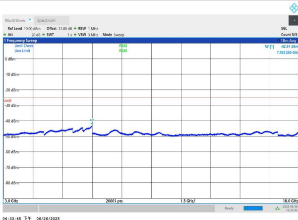
NTNV-n41-PC3-30-90-H-DFT-QPSK-Edge_1RB_Left-3000-1800 0-PASS
