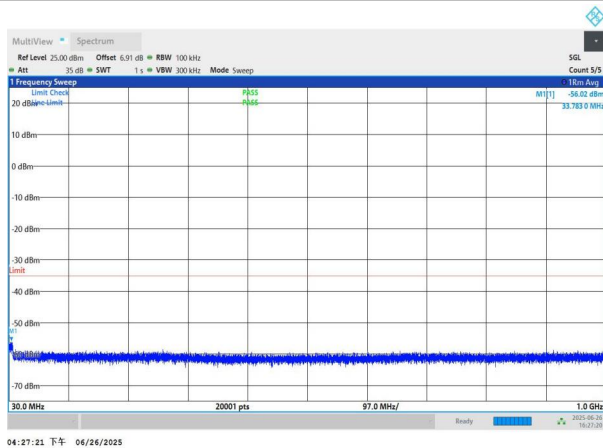
NTNV-n41-PC3-30-80-H-DFT-BPSK-Edge_1RB_Left-30-1000-P ASS
