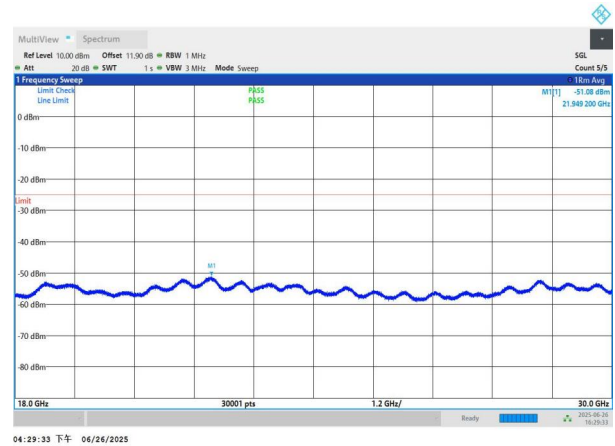
NTNV-n41-PC3-30-90-L-DFT-BPSK-Edge_1RB_Left-18000-3000
