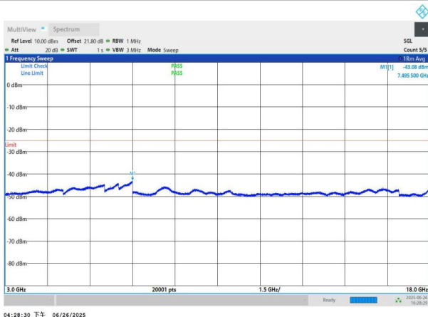
NTNV-n41-PC3-30-80-H-DFT-QPSK-Edge_1RB_Left-3000-1800 0-PASS
