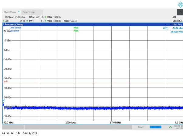
NTNV-n41-PC3-30-90-M-DFT-QPSK-Edge_1RB_Left-30-1000-P ASS
