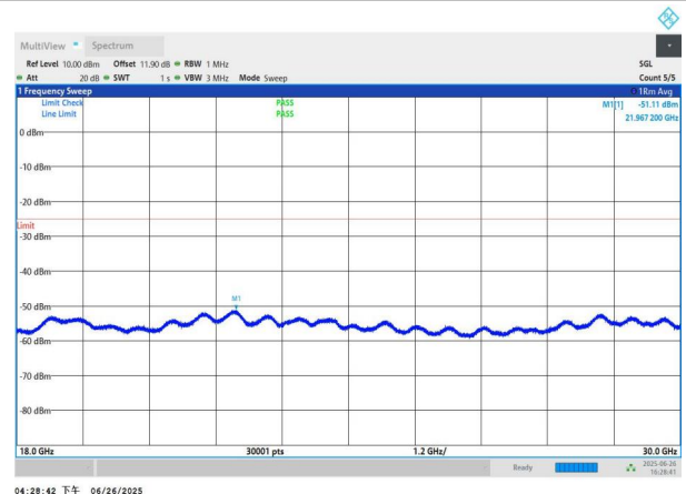
NTNV-n41-PC3-30-80-H-DFT-QPSK-Edge_1RB_Left-18000-3000 0-PASS
