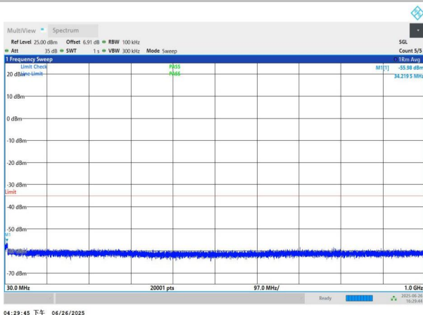
NTNV-n41-PC3-30-90-L-DFT-QPSK-Edge_1RB_Left-30-1000-PA
