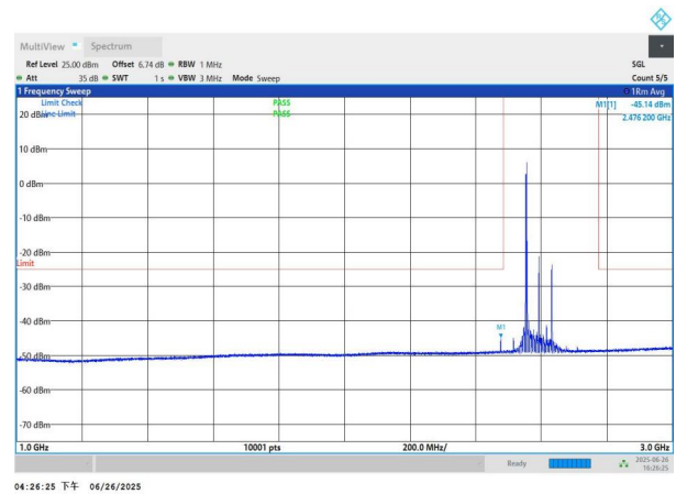
NTNV-n41-PC3-30-80-M-DFT-QPSK-Edge_1RB_Left-1000-3000- PASS
