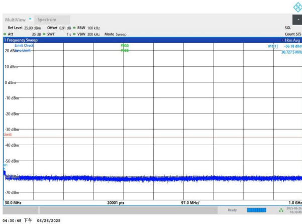
NTNV-n41-PC3-30-90-M-DFT-BPSK-Edge_1RB_Left-30-1000-P ASS
