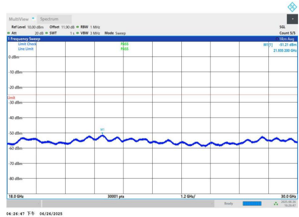
NTNV-n41-PC3-30-80-M-DFT-QPSK-Edge_1RB_Left-18000-3000 0-PASS
