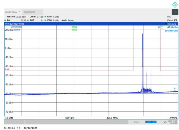
NTNV-n41-PC3-30-100-H-DFT-QPSK-Edge_1RB_Left-1000-3000- -PASS
