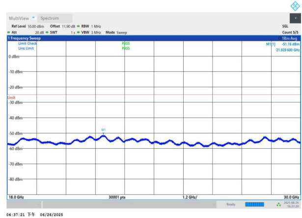
NTNV-n41-PC3-30-100-M-DFT-QPSK-Edge_1RB_Left-18000-300 00-PASS
