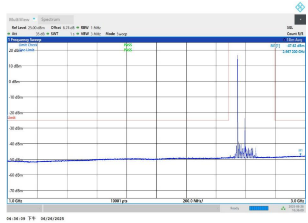
NTNV-n41-PC3-30-100-M-DFT-BPSK-Edge_1RB_Left-1000-3000- -PASS
