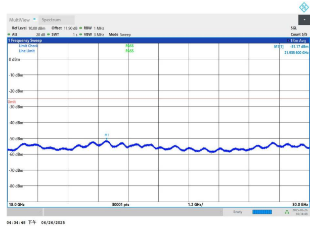
NTNV-n41-PC3-30-100-L-DFT-BPSK-Edge_1RB_Left-18000-300 00-PASS
