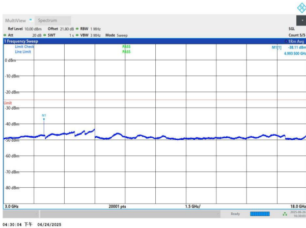
NTNV-n41-PC3-30-90-L-DFT-QPSK-Edge_1RB_Left-3000-1800 0-PASS
