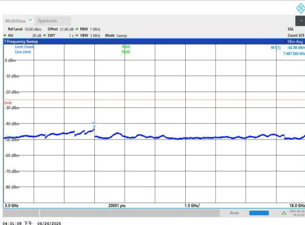
NTNV-n41-PC3-30-90-M-DFT-BPSK-Edge_1RB_Left-3000-1800 0-PASS
