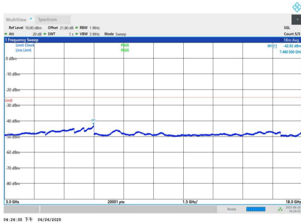
NTNV-n41-PC3-30-80-M-DFT-QPSK-Edge_1RB_Left-3000-1800 0-PASS
