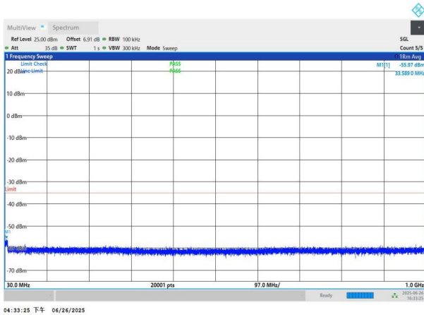
NTNV-n41-PC3-30-90-H-DFT-QPSK-Edge_1RB_Left-30-1000-P ASS
