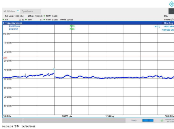
NTNV-n41-PC3-30-100-L-DFT-BPSK-Edge_1RB_Left-3000-1800 0-PASS
