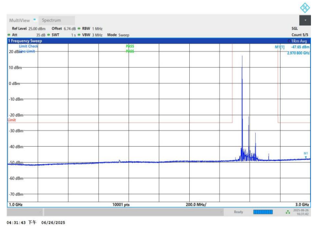
NTNV-n41-PC3-30-90-M-DFT-QPSK-Edge_1RB_Left-1000-3000- PASS
