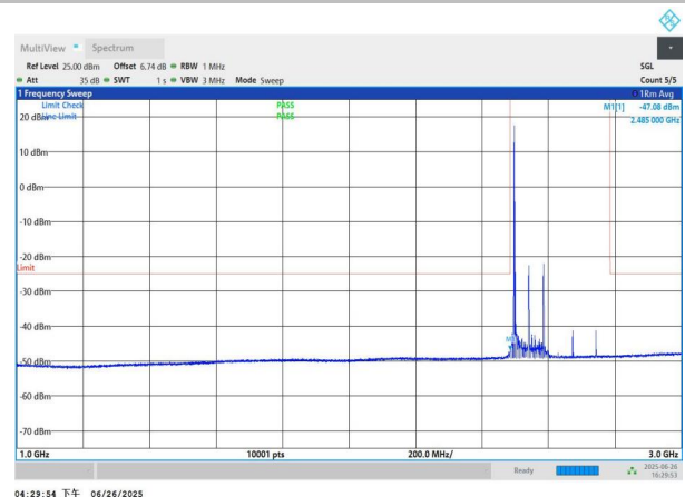
NTNV-n41-PC3-30-90-L-DFT-QPSK-Edge_1RB_Left-1000-3000-P
