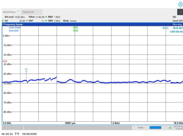
NTNV-n41-PC3-30-90-L-DFT-BPSK-Edge_1RB_Left-3000-18000
