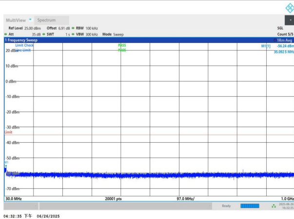
NTNV-n41-PC3-30-90-H-DFT-BPSK-Edge_1RB_Left-30-1000-P ASS
