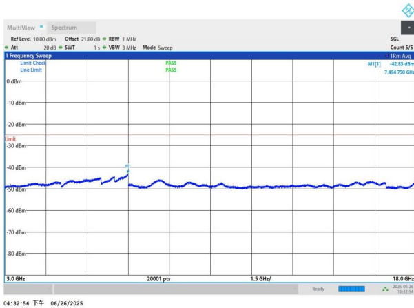
NTNV-n41-PC3-30-90-H-DFT-BPSK-Edge_1RB_Left-3000-1800 0-PASS
