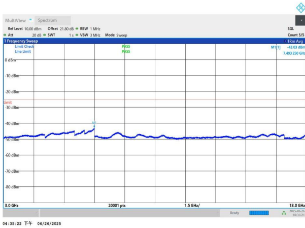
NTNV-n41-PC3-30-100-L-DFT-QPSK-Edge_1RB_Left-3000-180 00-PASS
