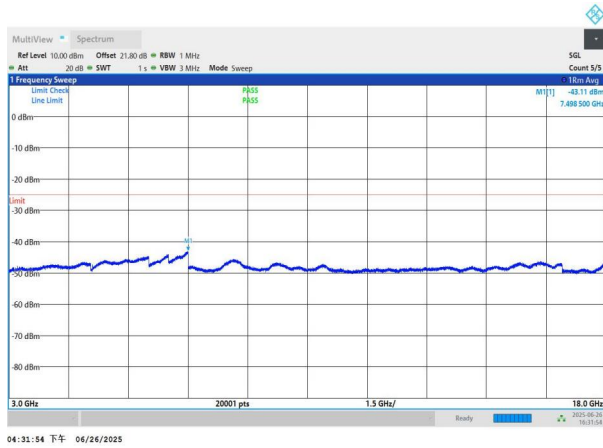
NTNV-n41-PC3-30-90-M-DFT-QPSK-Edge_1RB_Left-3000-1800 0-PASS
