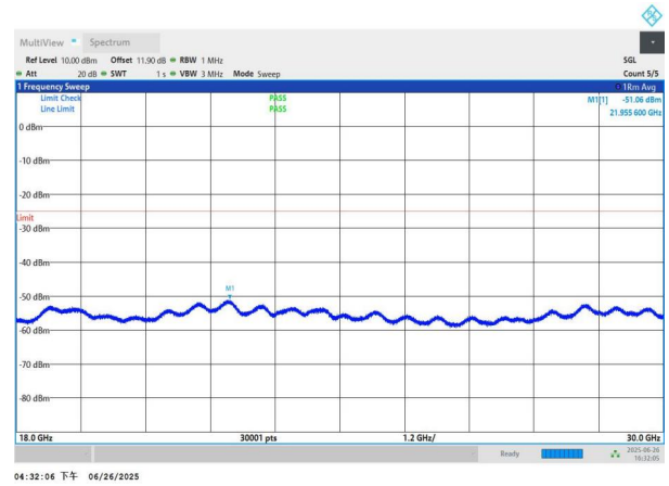
NTNV-n41-PC3-30-90-M-DFT-QPSK-Edge_1RB_Left-18000-3000 0-PASS
