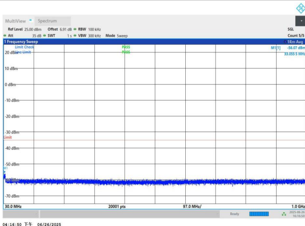
NTNV-n41-PC3-30-60-H-DFT-BPSK-Edge_1RB_Left-30-1000-P ASS
