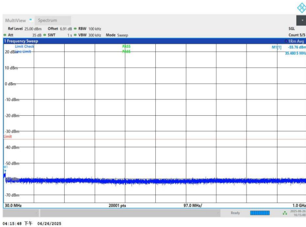
NTNV-n41-PC3-30-60-M-DFT-QPSK-Edge_1RB_Left-30-1000-P ASS
