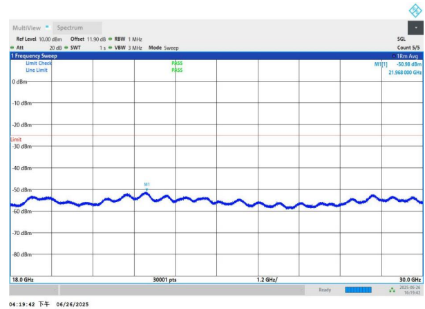
NTNV-n41-PC3-30-70-L-DFT-QPSK-Edge_1RB_Left-18000-3000 0-PASS
