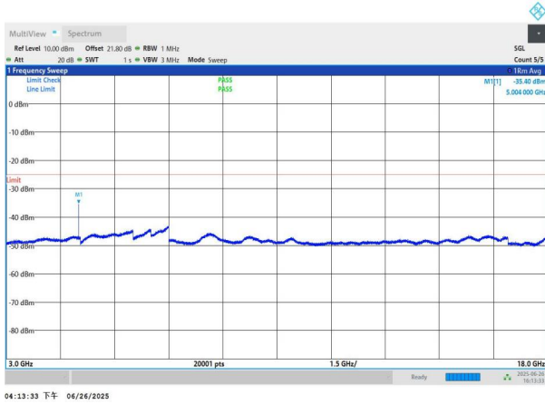
NTNV-n41-PC3-30-60-L-DFT-BPSK-Edge_1RB_Left-3000-18000
