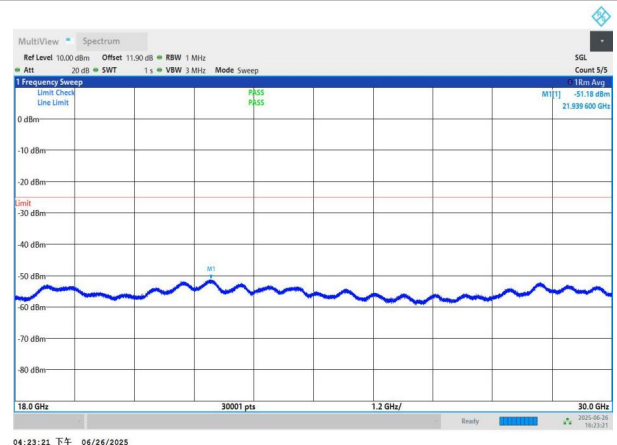
NTNV-n41-PC3-30-70-H-DFT-QPSK-Edge_1RB_Left-18000-3000 0-PASS
