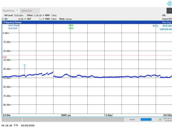
NTNV-n41-PC3-30-70-L-DFT-BPSK-Edge_1RB_Left-3000-18000 -PASS
