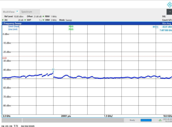
NTNV-n41-PC3-30-70-H-DFT-QPSK-Edge_1RB_Left-3000-1800 0-PASS
