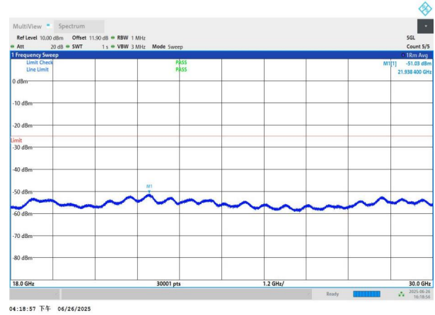
NTNV-n41-PC3-30-70-L-DFT-BPSK-Edge_1RB_Left-18000-3000 0-PASS
