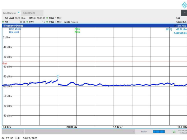
NTNV-n41-PC3-30-60-H-DFT-QPSK-Edge_1RB_Left-3000-1800 0-PASS
