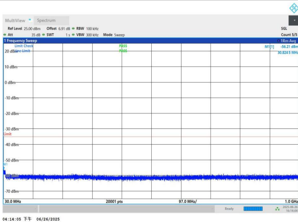
NTNV-n41-PC3-30-60-L-DFT-QPSK-Edge_1RB_Left-30-1000-PA
