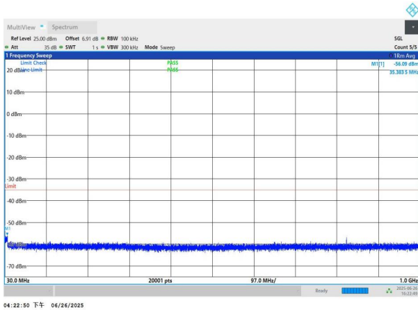
NTNV-n41-PC3-30-70-H-DFT-QPSK-Edge_1RB_Left-30-1000-P ASS
