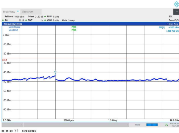
NTNV-n41-PC3-30-70-M-DFT-QPSK-Edge_1RB_Left-3000-1800 0-PASS
