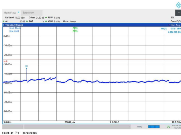
NTNV-n41-PC3-30-80-L-DFT-QPSK-Edge_1RB_Left-3000-1800 0-PASS
