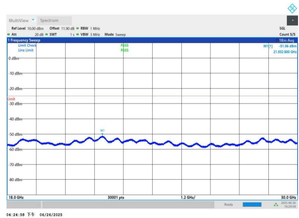
NTNV-n41-PC3-30-80-L-DFT-QPSK-Edge_1RB_Left-18000-3000 0-PASS
