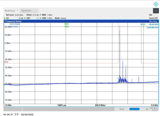
NTNV-n41-PC3-30-80-L-DFT-QPSK-Edge_1RB_Left-1000-3000-P ASS
