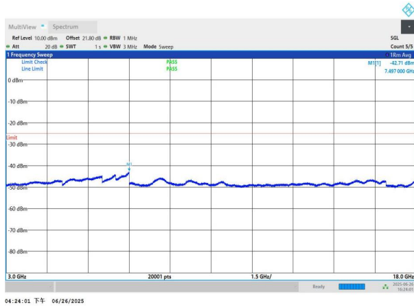
NTNV-n41-PC3-30-80-L-DFT-BPSK-Edge_1RB_Left-3000-18000 -PASS
