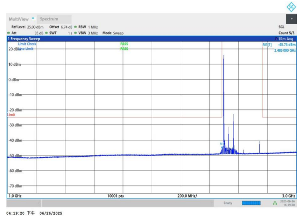
NTNV-n41-PC3-30-70-L-DFT-QPSK-Edge_1RB_Left-1000-3000-P ASS
