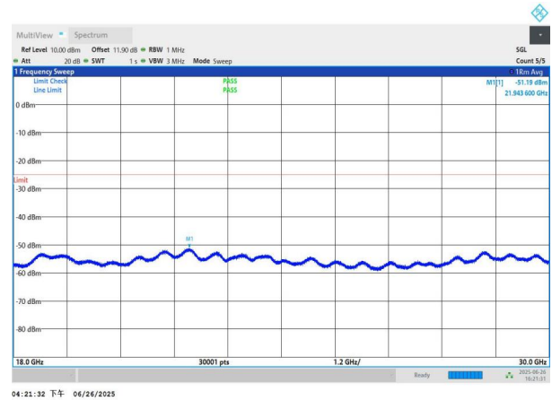
NTNV-n41-PC3-30-70-M-DFT-QPSK-Edge_1RB_Left-18000-3000 0-PASS
