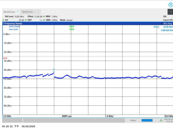
NTNV-n41-PC3-30-80-M-DFT-BPSK-Edge_1RB_Left-3000-1800 0-PASS
