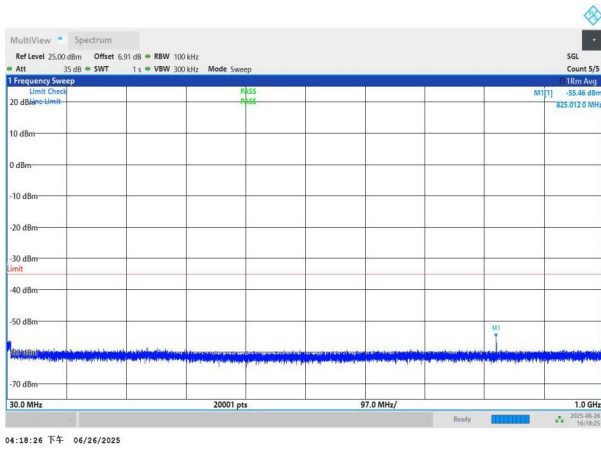
NTNV-n41-PC3-30-70-L-DFT-BPSK-Edge_1RB_Left-30-1000-PA SS
