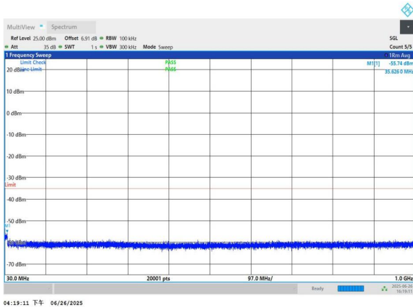
NTNV-n41-PC3-30-70-L-DFT-QPSK-Edge_1RB_Left-30-1000-PA SS
