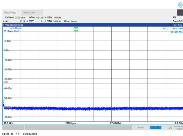
NTNV-n41-PC3-30-80-M-DFT-BPSK-Edge_1RB_Left-30-1000-P ASS
