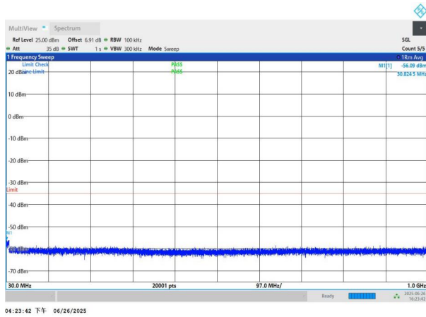
NTNV-n41-PC3-30-80-L-DFT-BPSK-Edge_1RB_Left-30-1000-PA SS
