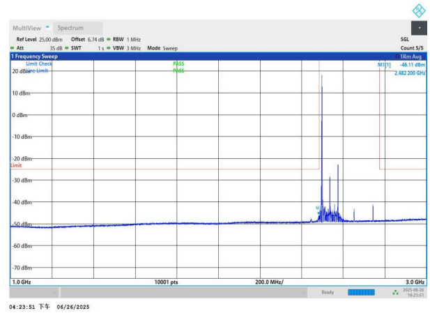
NTNV-n41-PC3-30-80-L-DFT-BPSK-Edge_1RB_Left-1000-3000-P ASS
