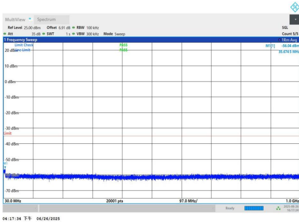
NTNV-n41-PC3-30-60-H-DFT-QPSK-Edge_1RB_Left-30-1000-P ASS
