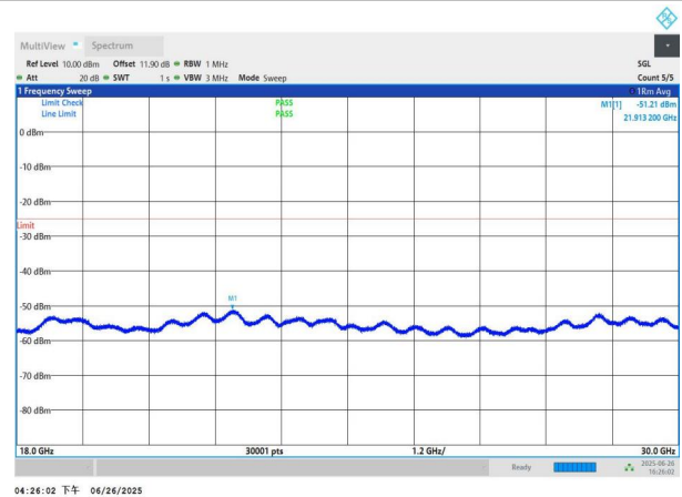
NTNV-n41-PC3-30-80-M-DFT-BPSK-Edge_1RB_Left-18000-3000 0-PASS
