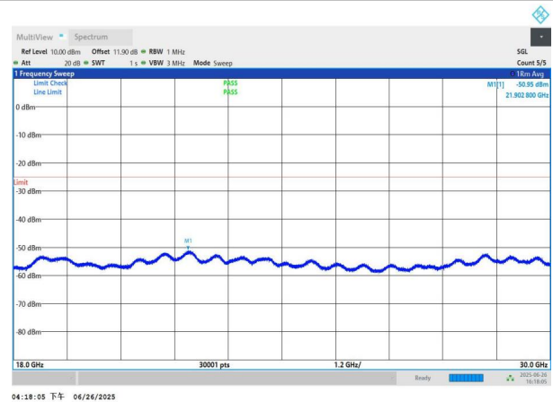
NTNV-n41-PC3-30-60-H-DFT-QPSK-Edge_1RB_Left-18000-3000 0-PASS
