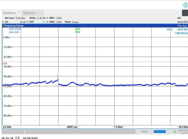
NTNV-n41-PC3-30-70-M-DFT-BPSK-Edge_1RB_Left-3000-1800 0-PASS
