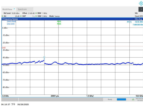
NTNV-n41-PC3-30-60-M-DFT-QPSK-Edge_1RB_Left-3000-1800 0-PASS
