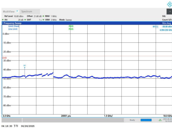
NTNV-n41-PC3-30-70-L-DFT-QPSK-Edge_1RB_Left-3000-1800 0-PASS
