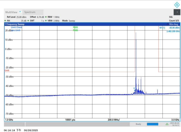
NTNV-n41-PC3-30-60-L-DFT-QPSK-Edge_1RB_Left-1000-3000-P
