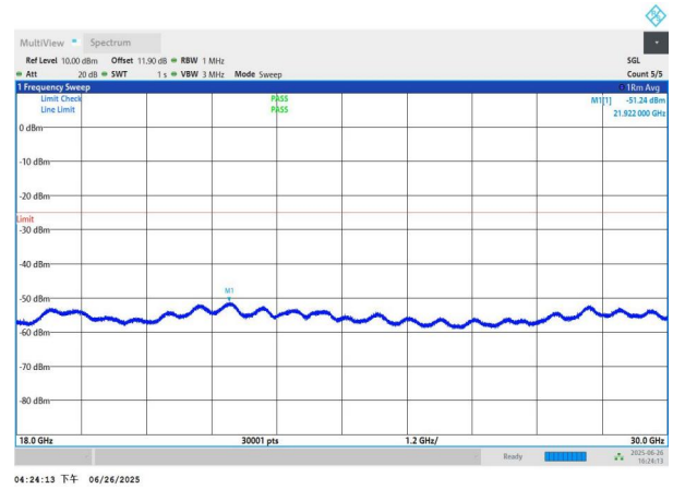
NTNV-n41-PC3-30-80-L-DFT-BPSK-Edge_1RB_Left-18000-3000 0-PASS
