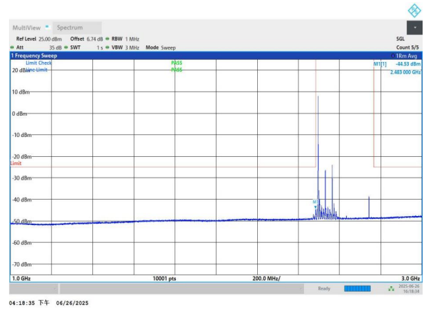
NTNV-n41-PC3-30-70-L-DFT-BPSK-Edge_1RB_Left-1000-3000-P ASS
