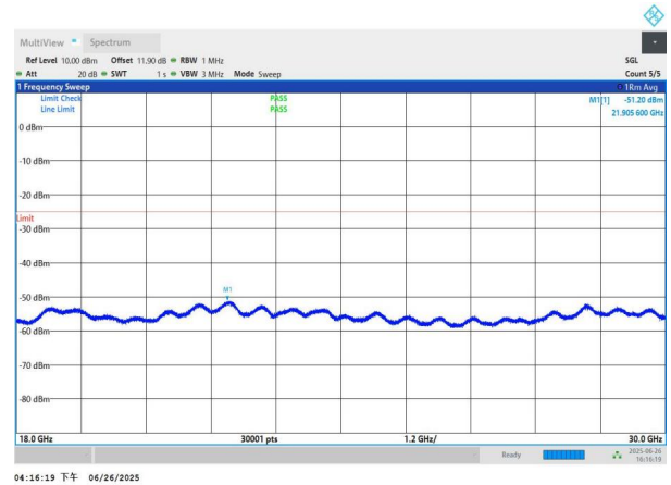
NTNV-n41-PC3-30-60-M-DFT-QPSK-Edge_1RB_Left-18000-3000 0-PASS
