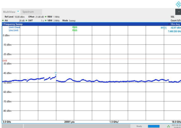
NTNV-n41-PC3-30-40-M-DFT-BPSK-Edge_1RB_Left-3000-1800 0-PASS
