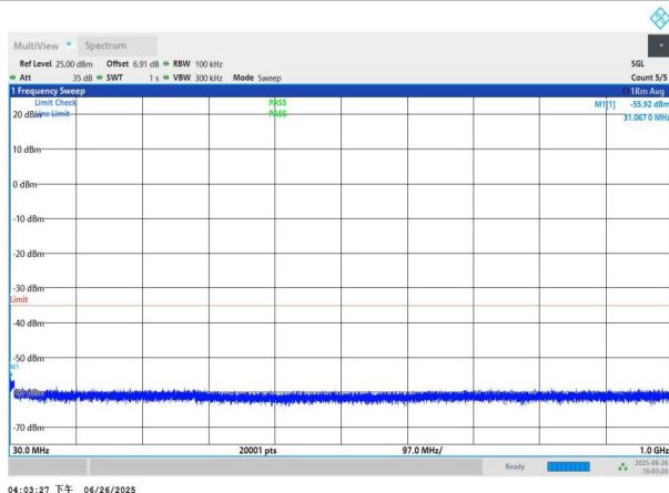
NTNV-n41-PC3-30-40-L-DFT-QPSK-Edge_1RB_Left-30-1000-PA SS
