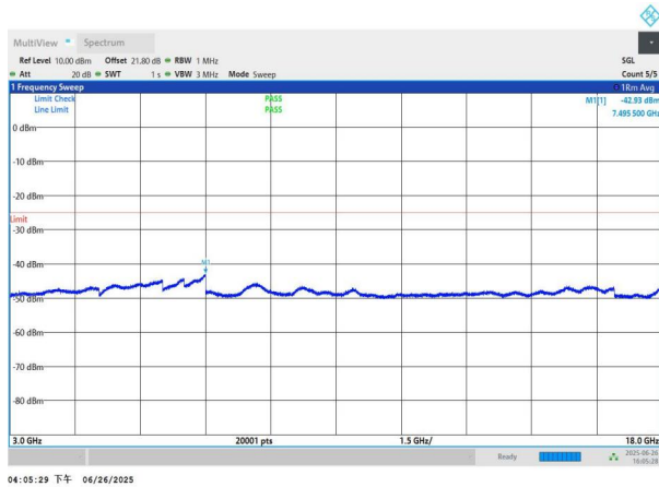
NTNV-n41-PC3-30-40-M-DFT-QPSK-Edge_1RB_Left-3000-1800 0-PASS
