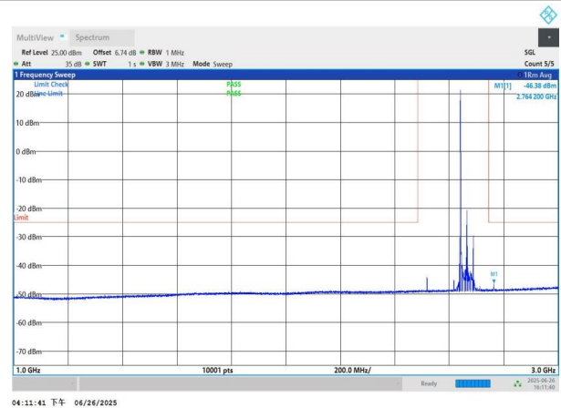
NTNV-n41-PC3-30-50-H-DFT-BPSK-Edge_1RB_Left-1000-3000-P ASS
