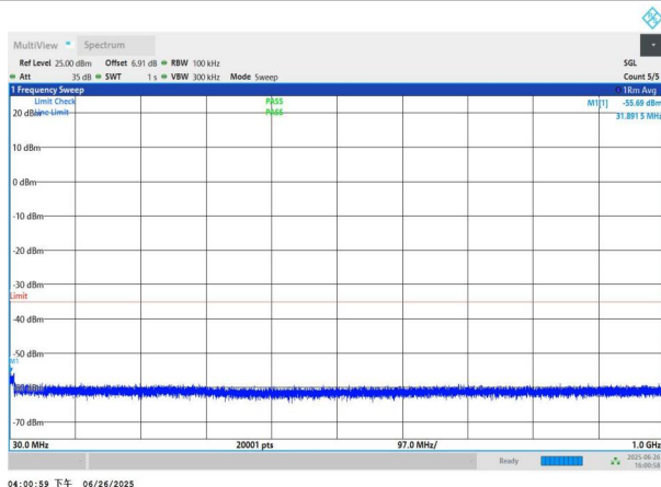
NTNV-n41-PC3-30-30-H-DFT-BPSK-Edge_1RB_Left-30-1000-P ASS
