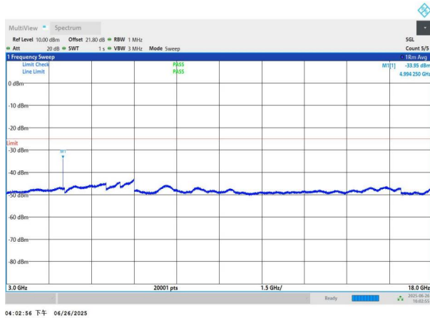
NTNV-n41-PC3-30-40-L-DFT-BPSK-Edge_1RB_Left-3000-18000 -PASS
