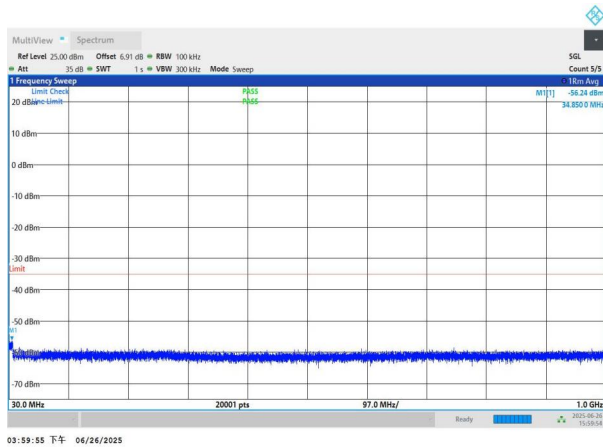
NTNV-n41-PC3-30-30-M-DFT-QPSK-Edge_1RB_Left-30-1000-P ASS
