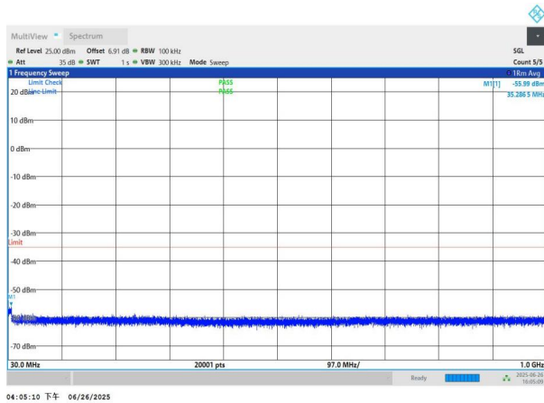
NTNV-n41-PC3-30-40-M-DFT-QPSK-Edge_1RB_Left-30-1000-P ASS
