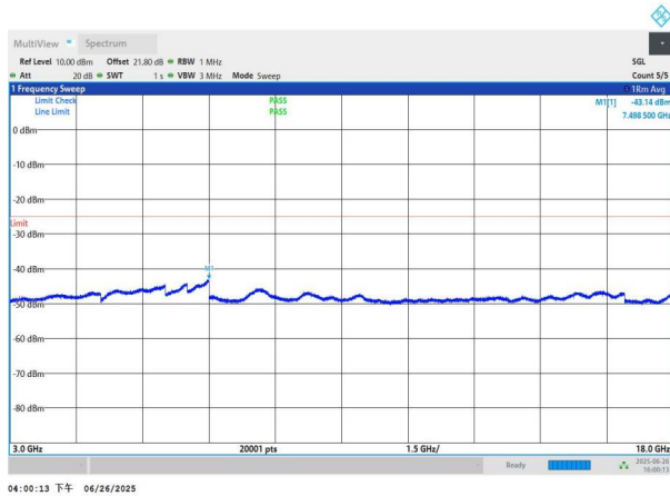
NTNV-n41-PC3-30-30-M-DFT-QPSK-Edge_1RB_Left-3000-1800 0-PASS
