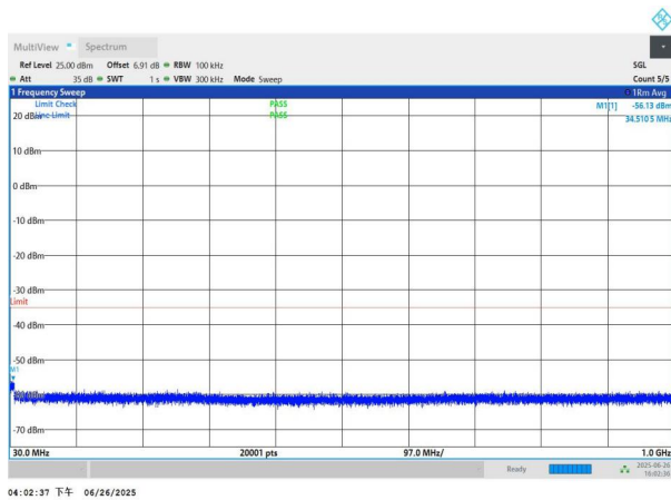
NTNV-n41-PC3-30-40-L-DFT-BPSK-Edge_1RB_Left-30-1000-PA SS
