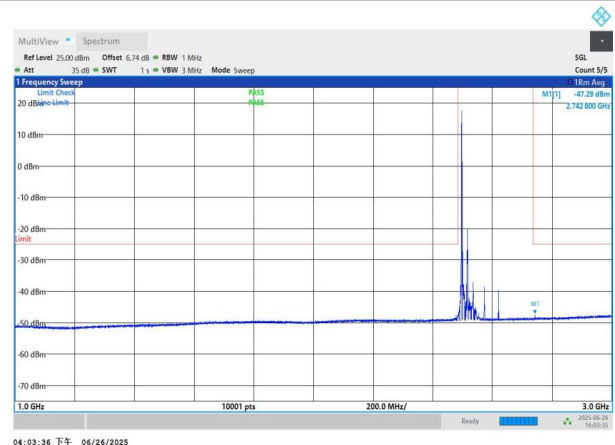
NTNV-n41-PC3-30-40-L-DFT-QPSK-Edge_1RB_Left-1000-3000-P ASS
