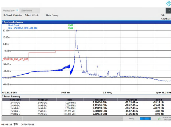
NTNV-n7-PC3-15-5-L-DFT-BPSK-Edge_1RB_Left-PASS
