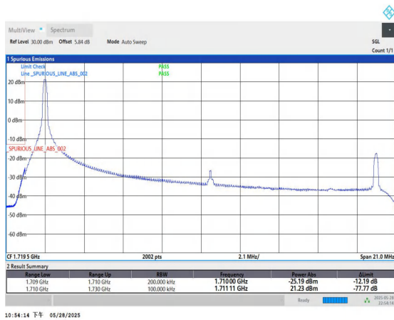
Band66-20MHz-QPSK-132072-1RB#0-PASS
