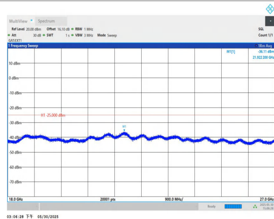
Band41-5MHz-QPSK-41565-1RB#0-18000~27000-PASS
