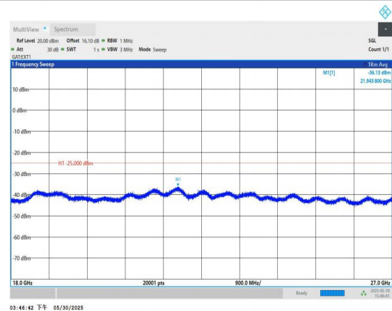
Band41-15MHz-QPSK-39725-1RB#0-18000~27000-PASS
