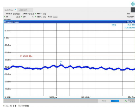
Band41-20MHz-QPSK-41490-1RB#0-18000~27000-PASS
