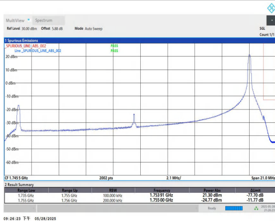
Band4-20MHz-QPSK-20300-1RB#99-PASS
