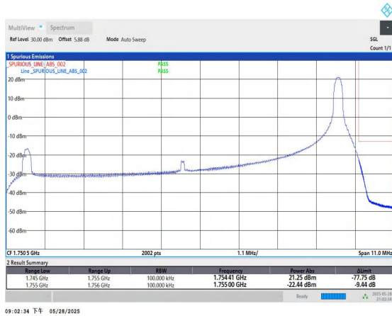
Band4-10MHz-QPSK-20350-1RB#49-PASS
