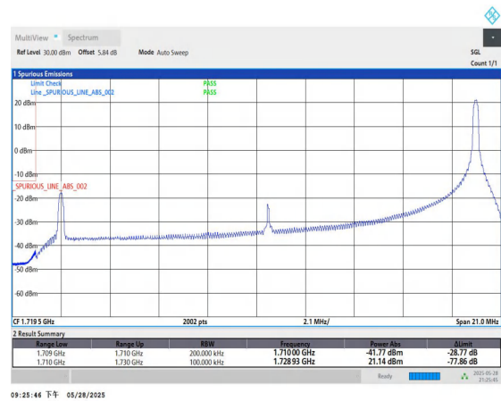
Band4-20MHz-QPSK-20050-1RB#99-PASS
