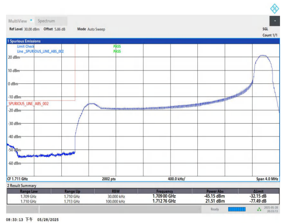
Band4-3MHz-QPSK-19965-1RB#14-PASS
