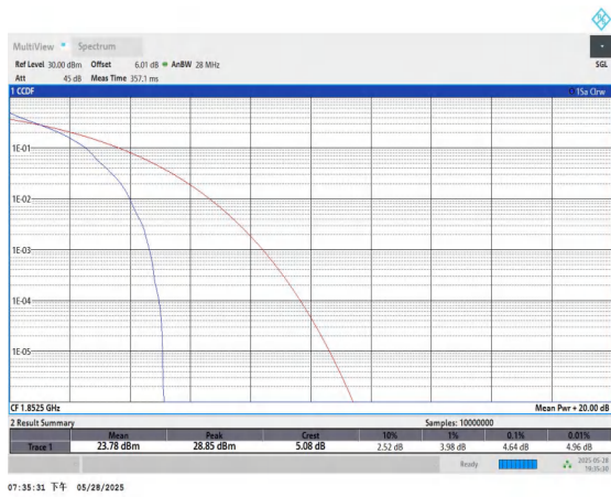
Band2-5MHz-QPSK-18625-1RB#0-PASS
