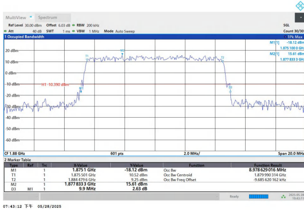
Band2-10MHz-16QAM-18900-50RB#0-PASS
