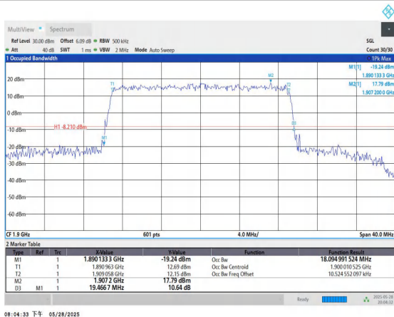
Band2-20MHz-QPSK-19100-100RB#0-PASS
