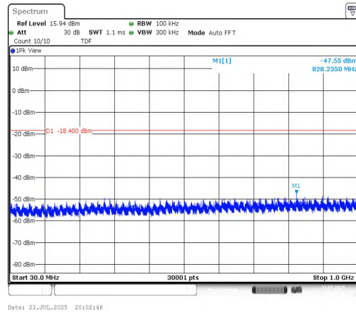
11G-Ant1-2437-30~1000-PASS
