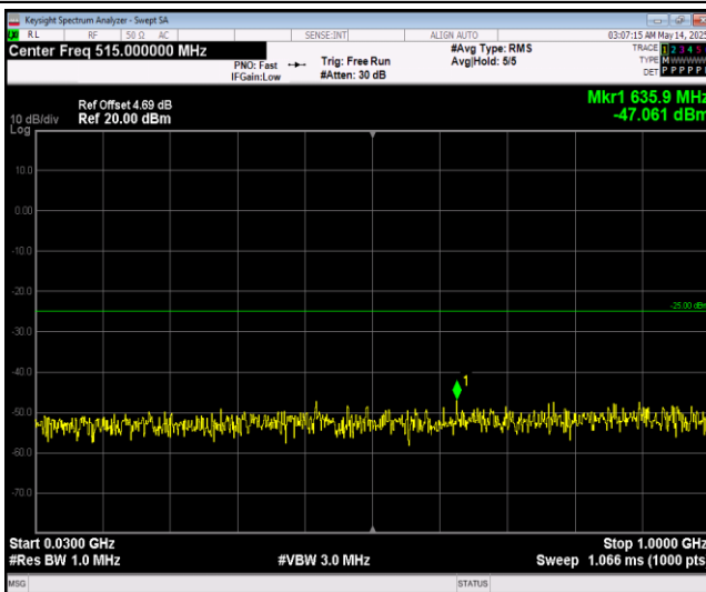
Band12-1.4MHz-QPSK-23017-1RB#0-Range1:30~1000MHz
