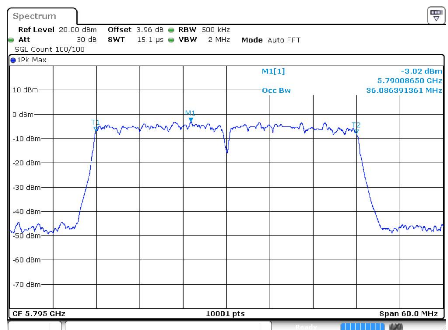
OBW n40 5795MHz Ant2
