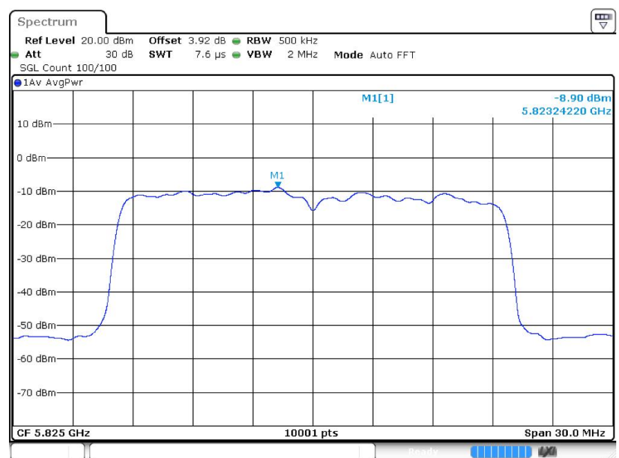
PSD ax20 5825MHz Ant1
