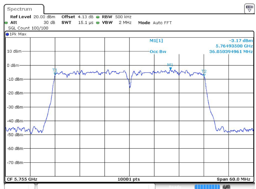
OBW n40 5755MHz Ant2
