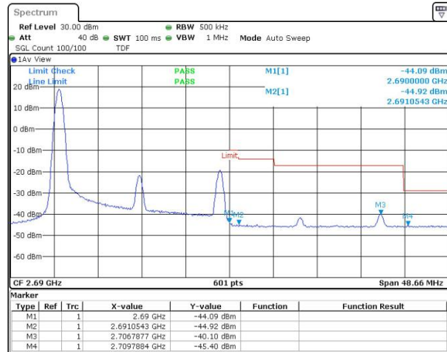
Band41-20MHz-QPSK-41490-1RB#99
