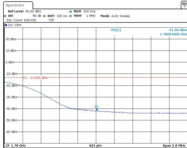
Band66-20MHz-QPSK-132572-1RB#99
