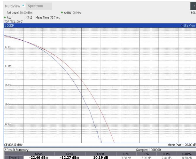
Band5-3MHz-QPSK-20635-1RB#0
