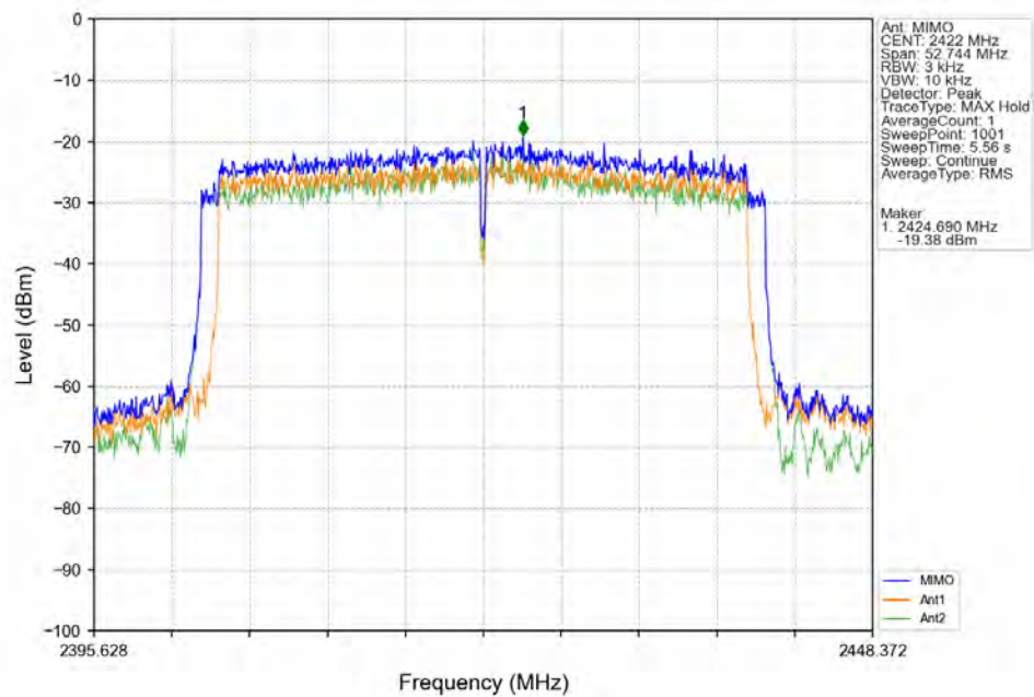
802.11ax(HEW40) LCH 2422MHz RU484 Left MIMO NTV
