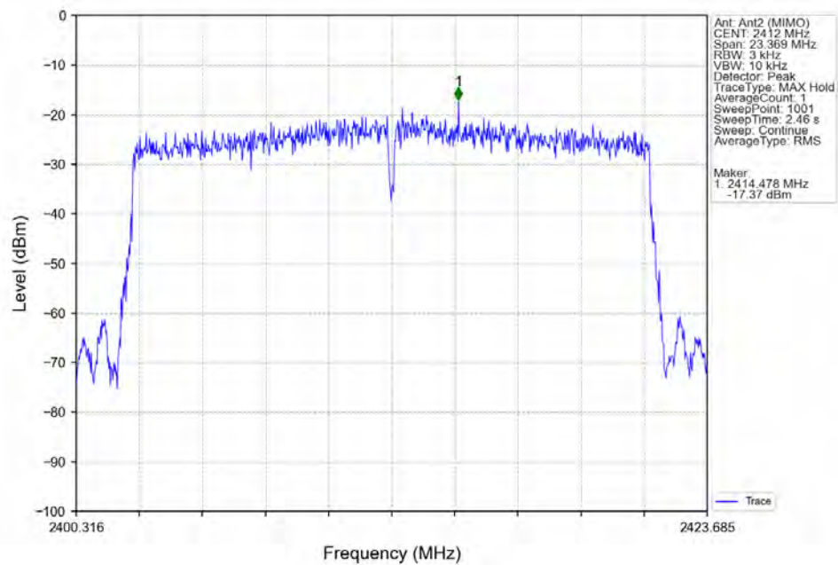
802.11ax(HEW20) LCH 2412MHz RU242 Left Ant2 (MIMO) NTVN
