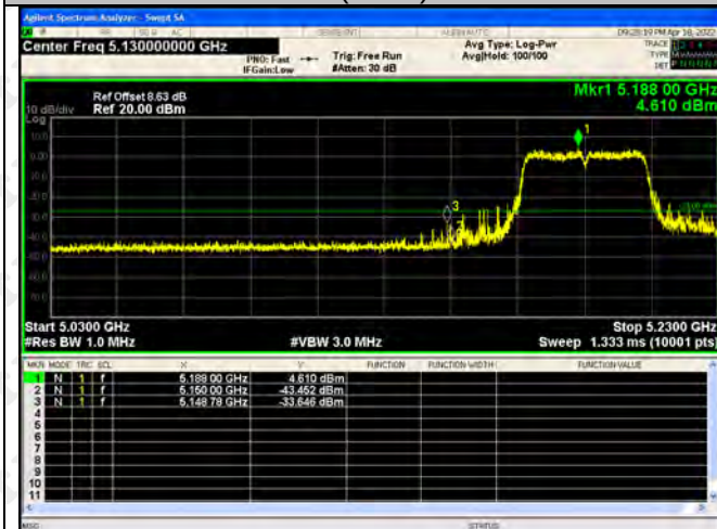
802.11ac(VH80)-5210
