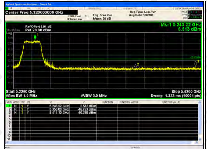
802.11n(HT40)-5230
