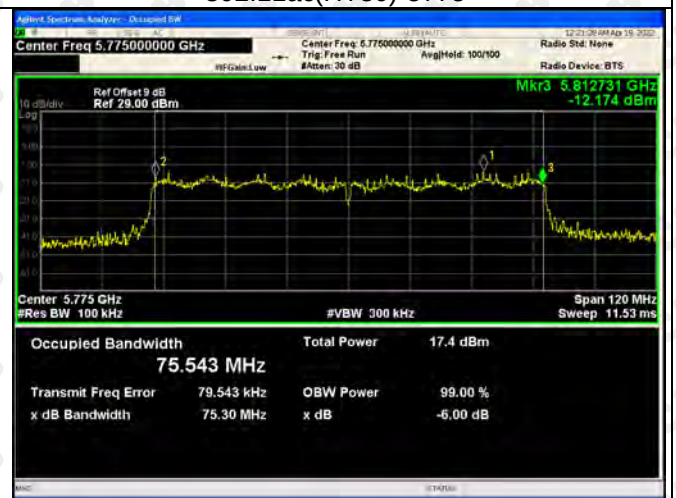
802.11ac(HT80)-5775
