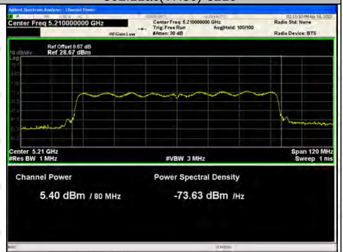
802.11ac(VH80)-5210
