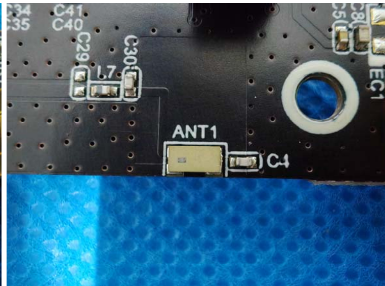
Antenna
