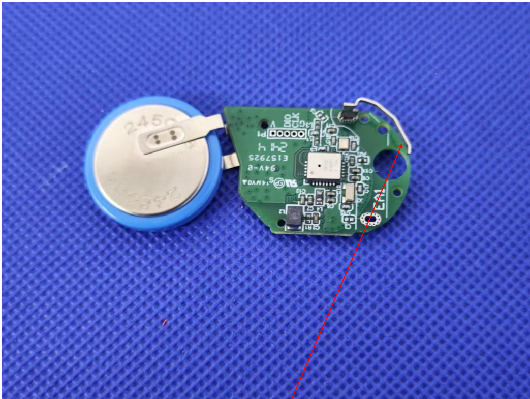
ANTANNA
