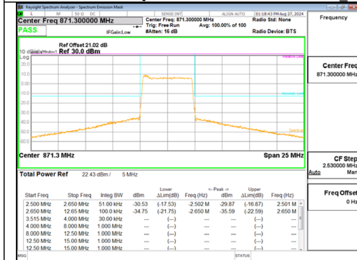
5G NR N26(22H) QPSK 5M RB25-0 Low Ch – BTS 3
