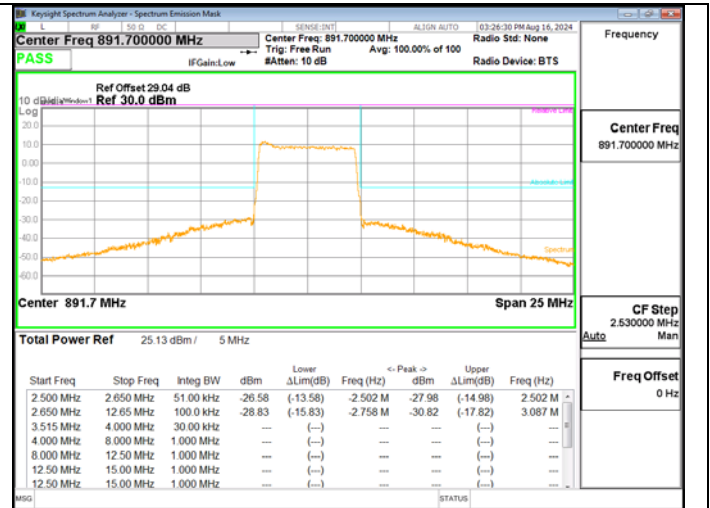
5G NR N26(22H) QPSK 5M RB25-0 High Ch – BTS 1
