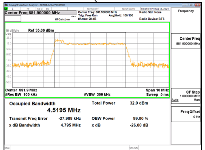
5G NR n26 (22H) QPSK Mid Channel
