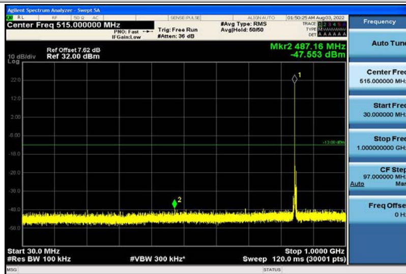
Band5-3MHz-QPSK-20635-1RB#0-30~1000MHz
