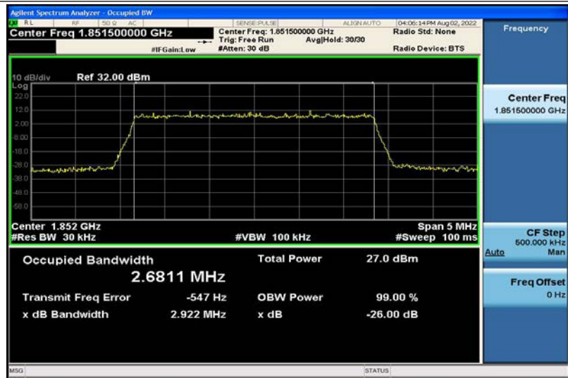
Band2-3MHz-QPSK-18615-15RB#0-2.6811
