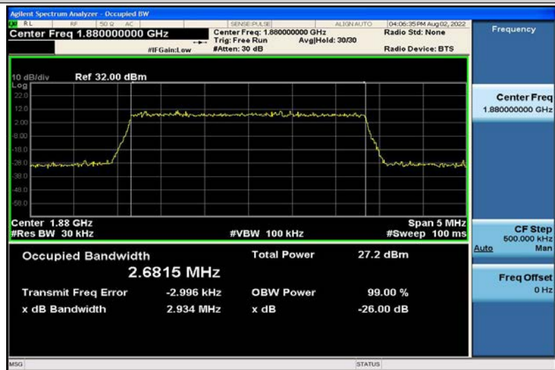
Band2-3MHz-QPSK-18900-15RB#0-2.6815
