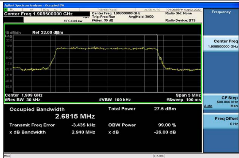
Band2-3MHz-QPSK-19185-15RB#0-2.6815
