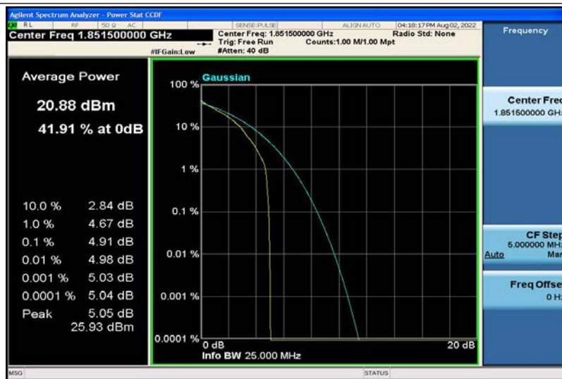
Band2-3MHz-QPSK-18615-1RB#0
