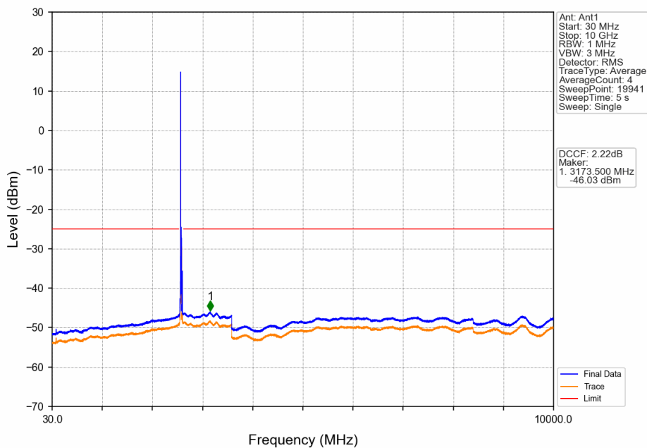
Band38_20MHz_16QAM_MCH_2595MHz_RB_1_0_NTNV
