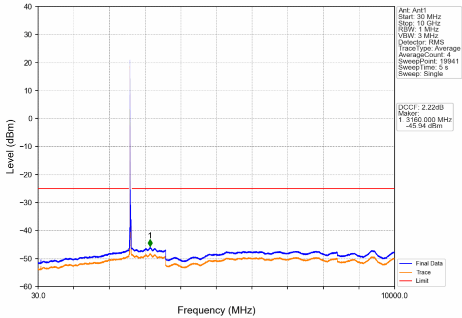
Band38 20MHz QPSK HCH 2610MHz RB 1_0 NTN
