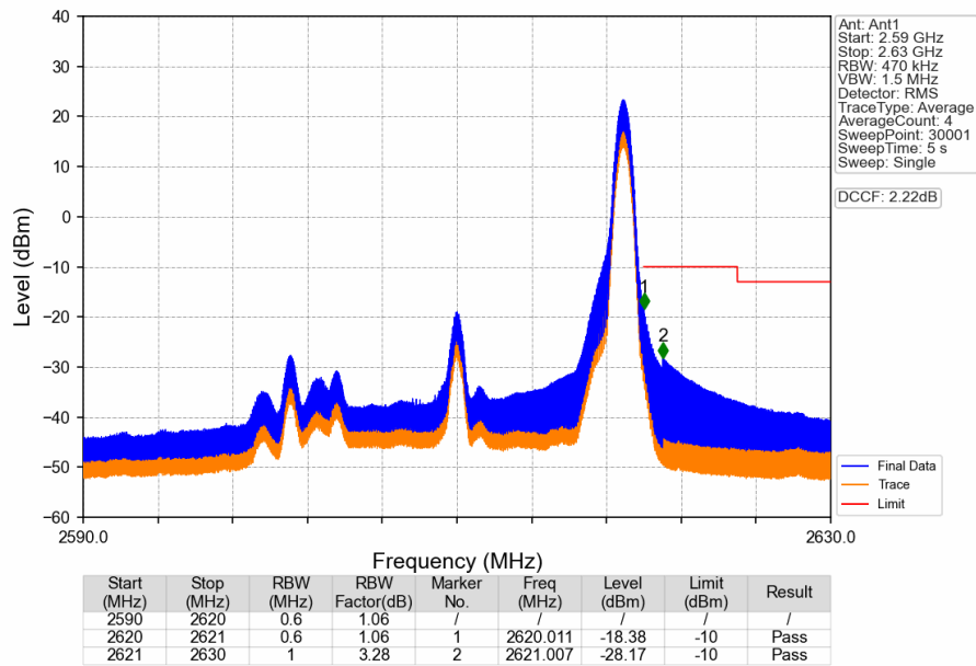
Band38_20MHz_QPSK_HCH_2610MHz_RB_1_99_NTNV
