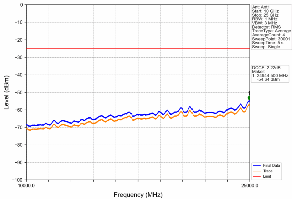
Band38 20MHz QPSK HCH 2610MHz RB 1_0 NTN
