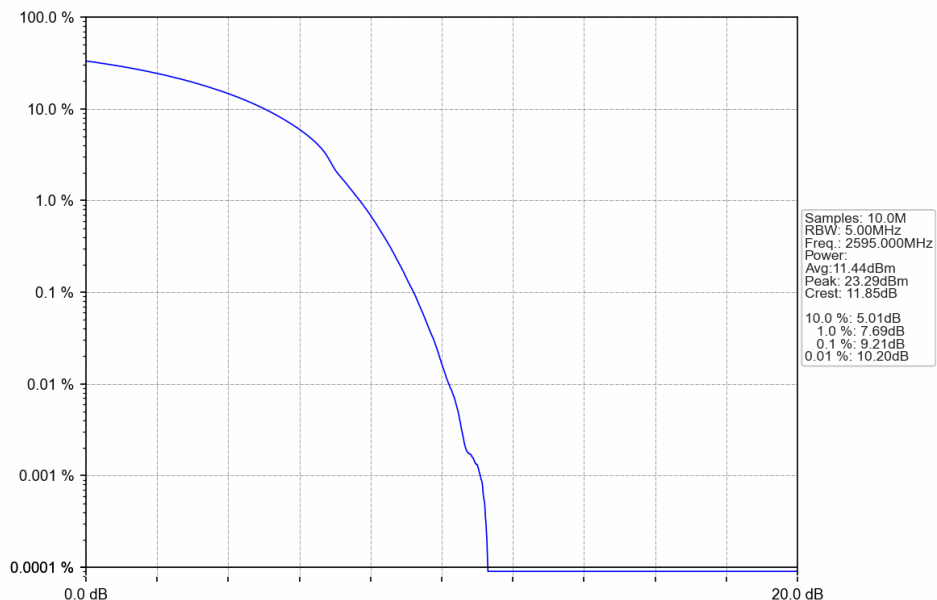
Band38_20MHz_16QAM_MCH_2595MHz_RB_100_0_NTNV
