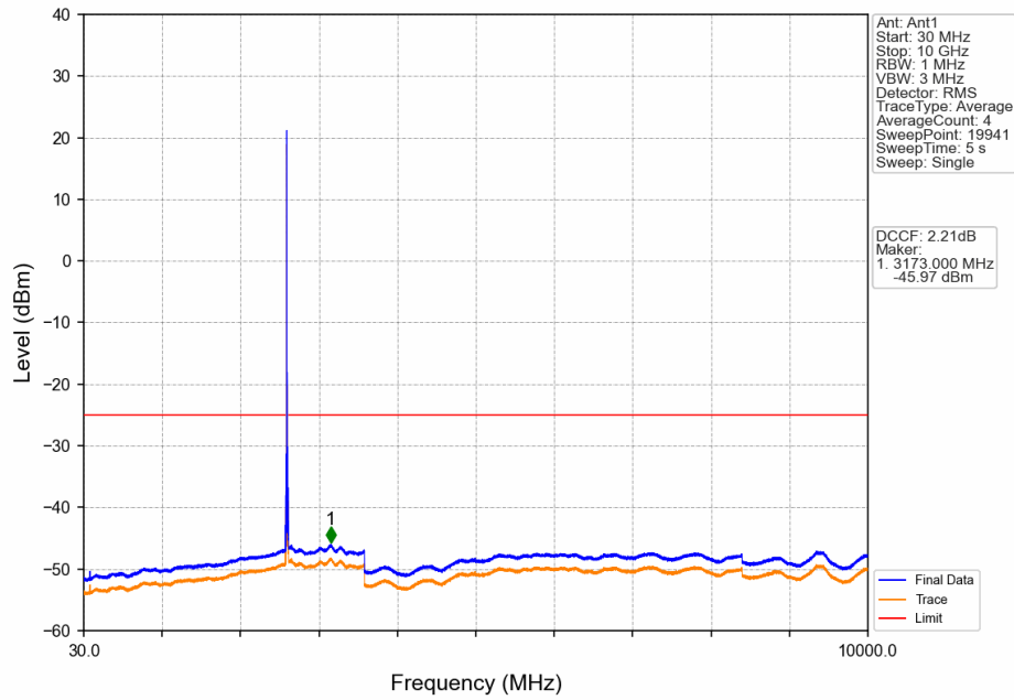
Band38_10MHz_QPSK_HCH_2615MHz_RB_1_0_NTNV
